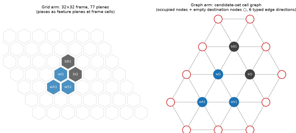
Fig. 3 — Les deux encodages d’une même position : plans en grille dans le cadre 32×32 (gauche) et graphe de cellules avec ses six relations typées par direction (droite).
