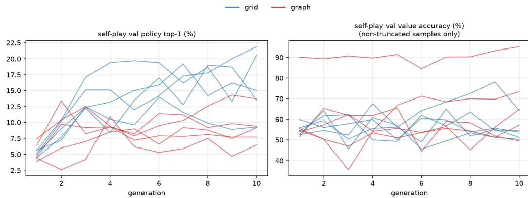
Fig. 6 — Métriques d'entraînement par génération (top-1 politique et exactitude valeur à l'époque 1, 10 exécutions de la campagne principale ; exécutions d'ablation exclues).
