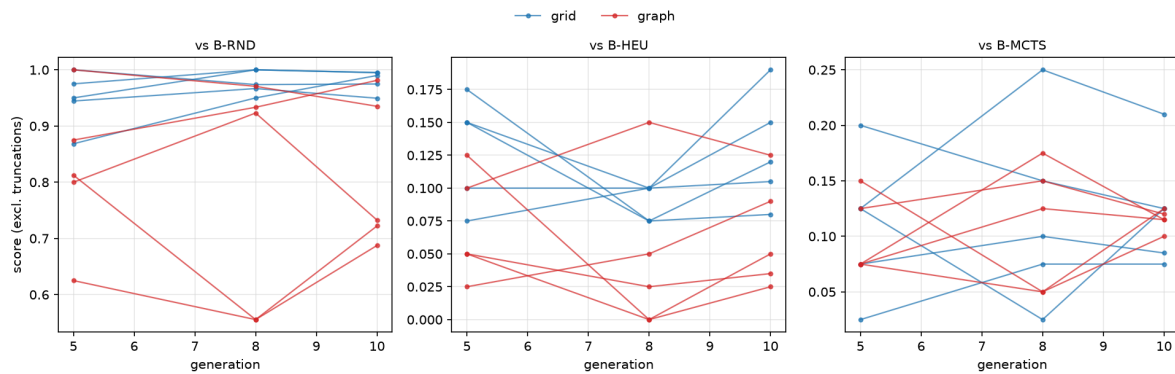
Fig. 9 : Score contre chaque adversaire gelé aux générations évaluées (5, 8 et 10 ; 20, 20 et 100 parties par adversaire respectivement) pour chaque exécution principale. Bleu : bras grille ; rouge : bras graphe ; une ligne par graine. Les scores excluent les parties tronquées.
