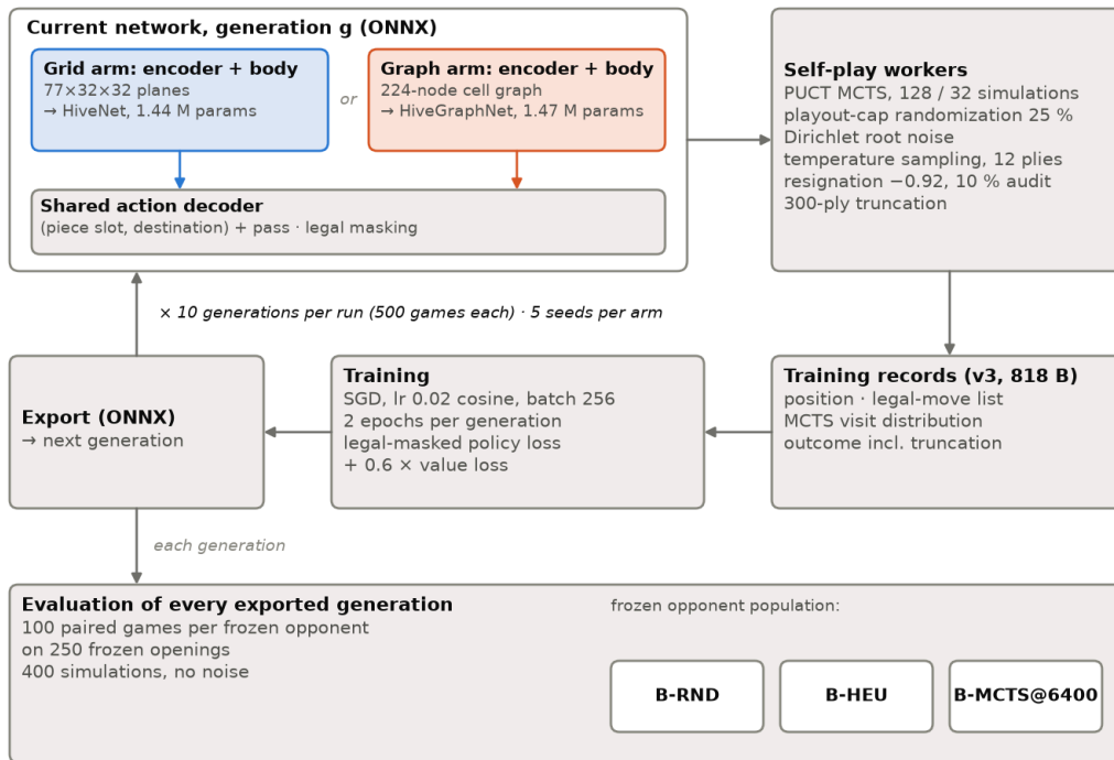
Fig. 3 : La boucle de générations partagée par les deux bras. L'auto-jeu avec recherche arborescente Monte-Carlo produit des enregistrements d'entraînement ; les enregistrements entraînent un réseau ; le réseau est exporté en ONNX et pilote l'auto-jeu de la génération suivante ; à des générations fixées, le réseau exporté est évalué contre la population d'adversaires gelée (B-RND, B-HEU, B-MCTS) sur des ouvertures gelées. Le bras grille et le bras graphe ne diffèrent que par l'encodeur d'état et le corps du réseau à l'intérieur des boîtes marquées « réseau ».
