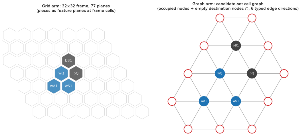
Fig. 1 : Une position de Hive à cinq tuiles sous les deux encodages comparés dans cette étude. À gauche, la vue du bras grille : la position plongée dans un cadre fixe 32×32 de cellules hexagonales (dessinées pour l'orientation), chaque cellule du cadre portant 77 valeurs de caractéristiques, de sorte que les tuiles apparaissent comme des activations aux coordonnées du cadre. À droite, la vue du bras graphe : le graphe de cellules sur l'ensemble candidat, dans lequel les cellules occupées (pleines, étiquetées par couleur et par tuile) et chaque cellule vide adjacente à la ruche (cercles ouverts), formant ensemble l'ensemble de toutes les destinations légales, sont reliées par des arêtes typées par les six directions hexagonales. Les deux vues dérivent du même état du moteur sans perte ; seule la structure offerte au réseau diffère.
