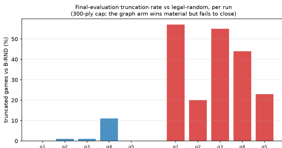
Fig. 7 : Taux de troncature à l'évaluation finale contre l'adversaire aléatoire légal pour chacune des dix exécutions principales (points de contrôle finaux ; 100 parties par exécution à 400 simulations sur les 250 ouvertures gelées ; plafond de 300 plis). Bleu : bras grille, graines 1–5 ; rouge : bras graphe, graines 1–5. La troncature est rapportée séparément des nulles tout au long de l'étude.
