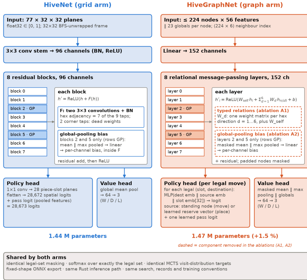
Fig. 4 : Schémas par blocs des deux réseaux. À gauche, HiveNet (bras grille) : tronc convolutif 3 \times 3 , 8 blocs résiduels de 96 canaux avec un biais de pooling global dans les blocs 2 et 5, une tête de politique plate à 28 673 sorties et une tête de valeur à 3 classes, 1.44 M paramètres au total. À droite, HiveGraphNet (bras graphe) : couche linéaire d'entrée vers 152 canaux, 8 couches relationnelles à passage de messages avec six matrices typées par direction et un biais de pooling global une couche sur trois, une fonction de notation de politique par candidat sur les plongements de destination, de source et d'emplacement, et une tête de valeur moyenne \parallel max masquée, 1.47 M paramètres au total. Les deux réseaux alimentent le décodeur d'actions partagé ; seuls l'encodeur et le corps diffèrent.
