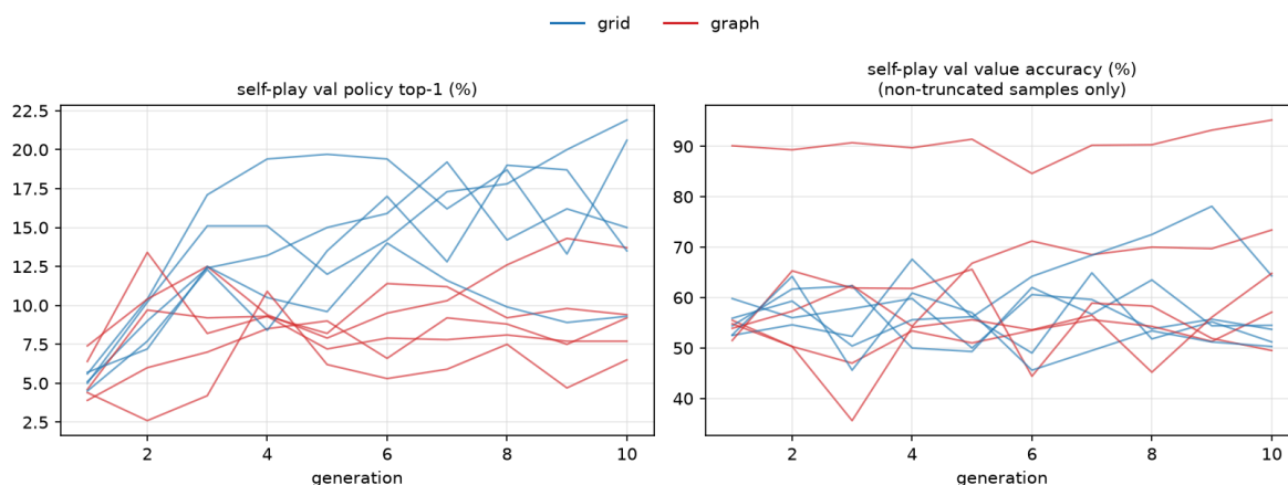
Fig. 8 : Métriques d'entraînement par génération pour les dix exécutions de la campagne principale (ligne de l'époque 1 de chaque génération) : à gauche, accord top-1 de la politique avec la distribution de visites MCTS sur la partition de validation d'auto-jeu ; à droite, exactitude de la valeur sur les échantillons non tronqués. Bleu : bras grille ; rouge : bras graphe ; une ligne par graine. Les exécutions d'ablation sont exclues.
