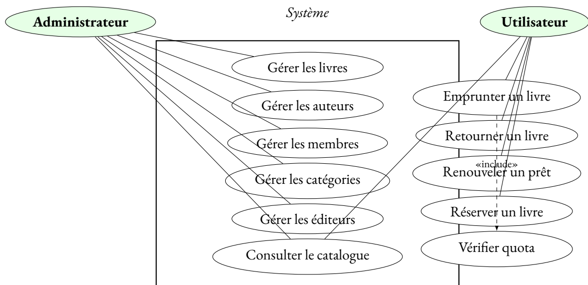
FIGURE 2.2 – Diagramme de cas d'utilisation
