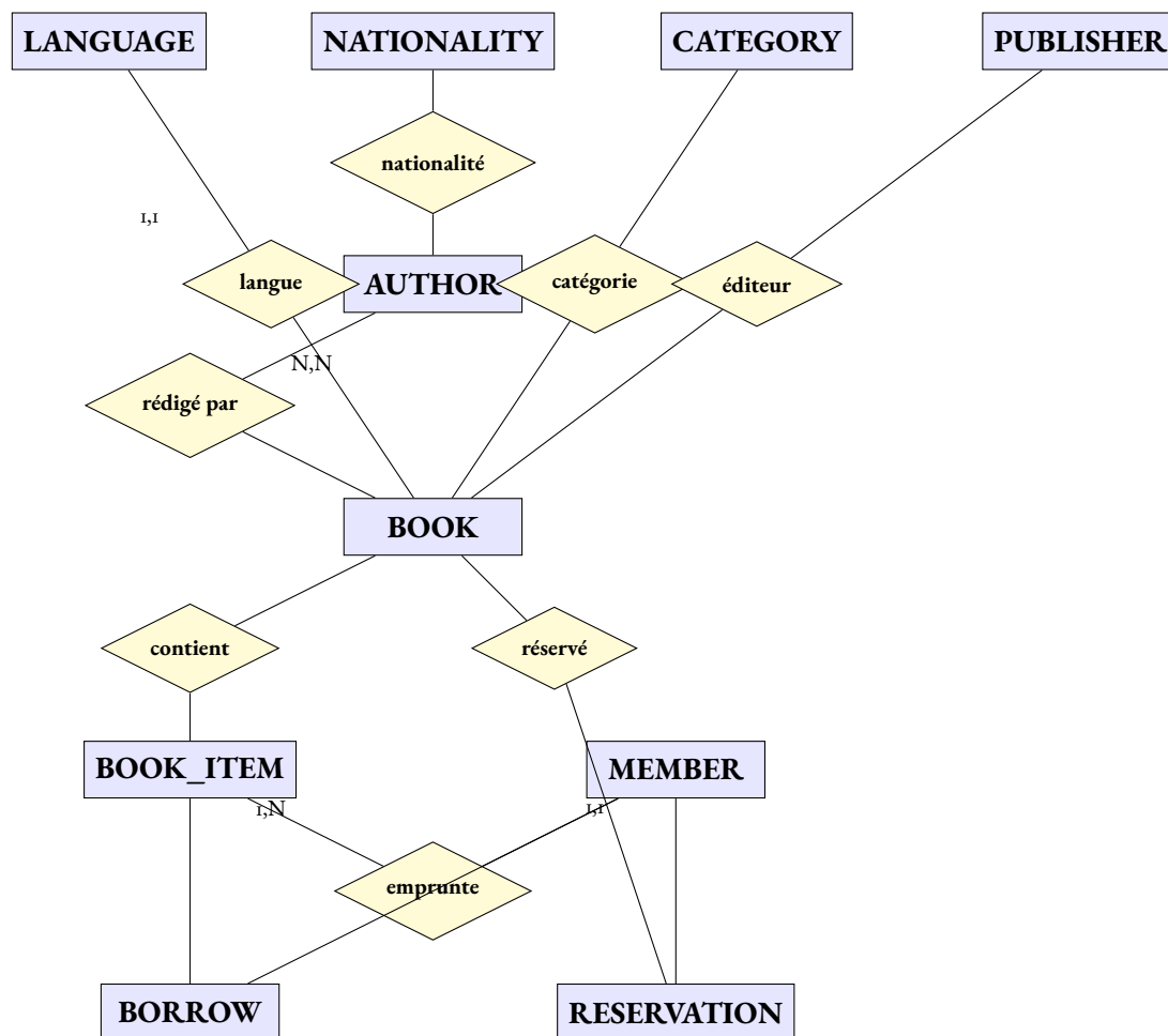
FIGURE 2.1 – Modèle Conceptuel de Données du système
