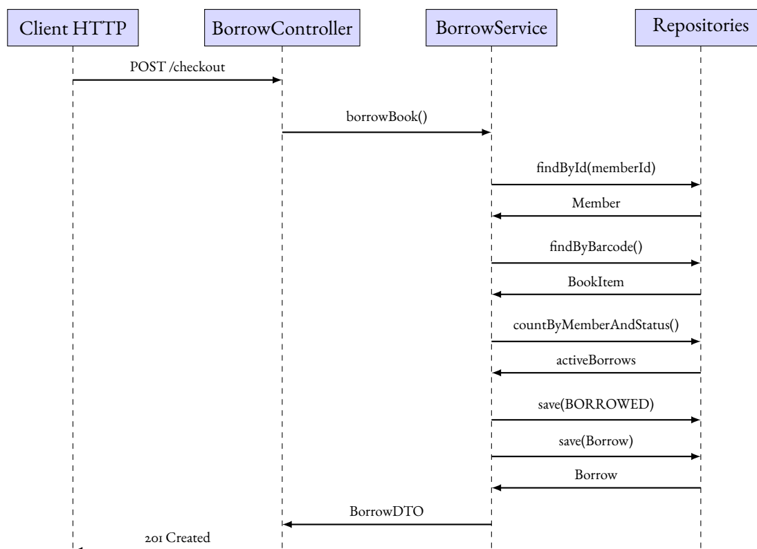
FIGURE 2.3 – Diagramme de séquence - Emprunt d'un livre
