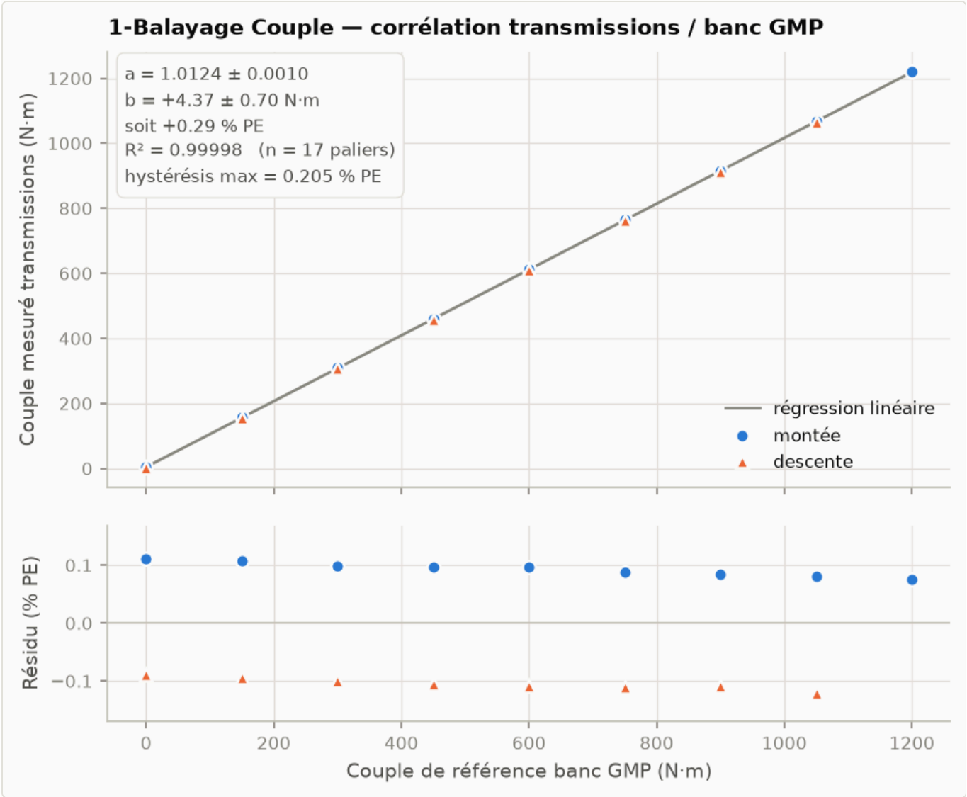
Exemple de figure produite : régression du balayage couple, avec le panneau des résidus. Écrite en PNG dans le dossier de sortie, prête pour le rapport.
