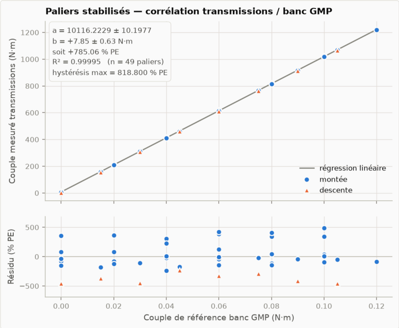
Exemple de figure produite : régression sur les paliers stabilisés de toute la campagne, avec le panneau des résidus. Écrite en PNG dans le dossier de sortie, prête pour le rapport.
