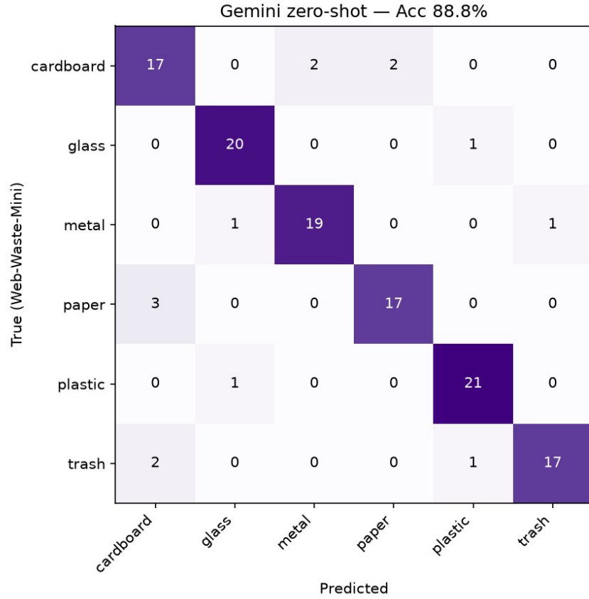
شكل (4-5): مصفوفة الالتباس لـ Gemini Vision
