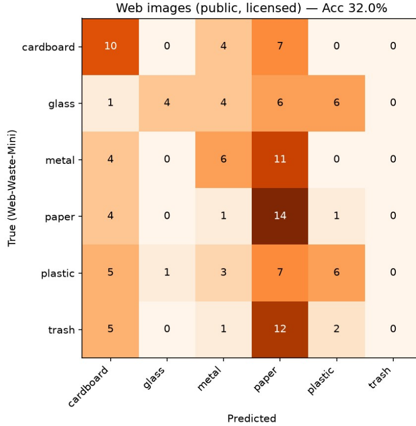
شكل (3-5): مصفوفة الالتباس الخارجية (Web-Waste-Mini)
