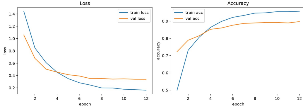
شكل (5-1): منحني التدريب
