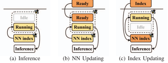
Fig. 4: Parameter hot-updating
