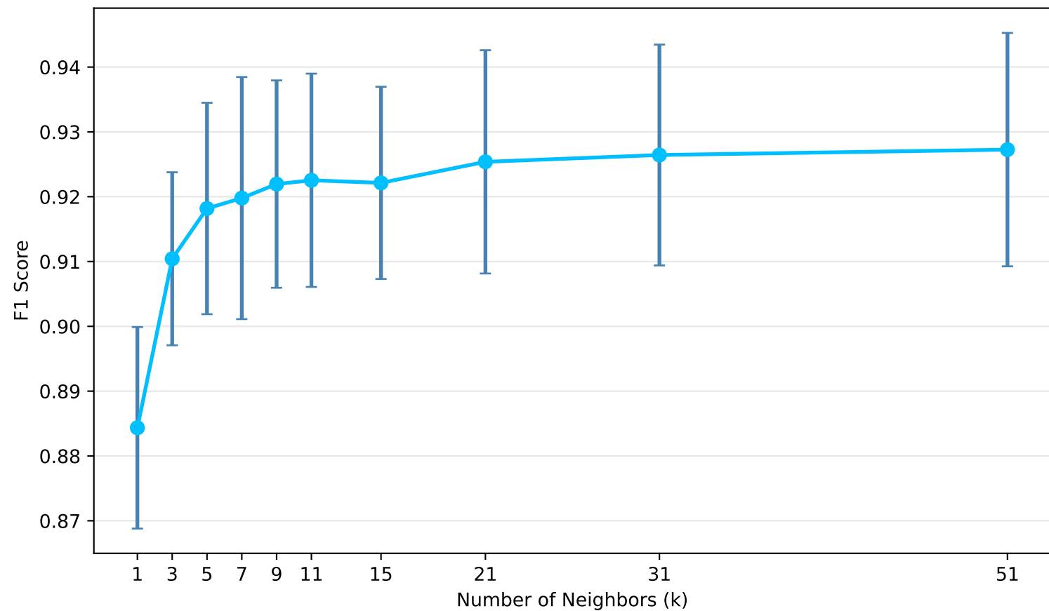
Dataset 1.3 (Rice): F1 Score vs. k
