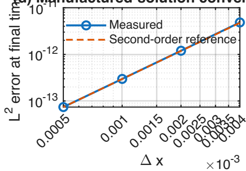
(d) Manufactured-solution convergence
