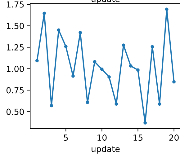
entropy (nats/token)
