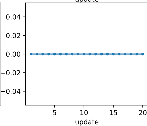
clip fraction
