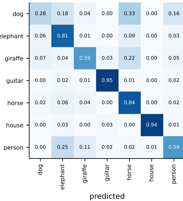
DAN-DG ( \lambda=1 ) (acc 0.687)
