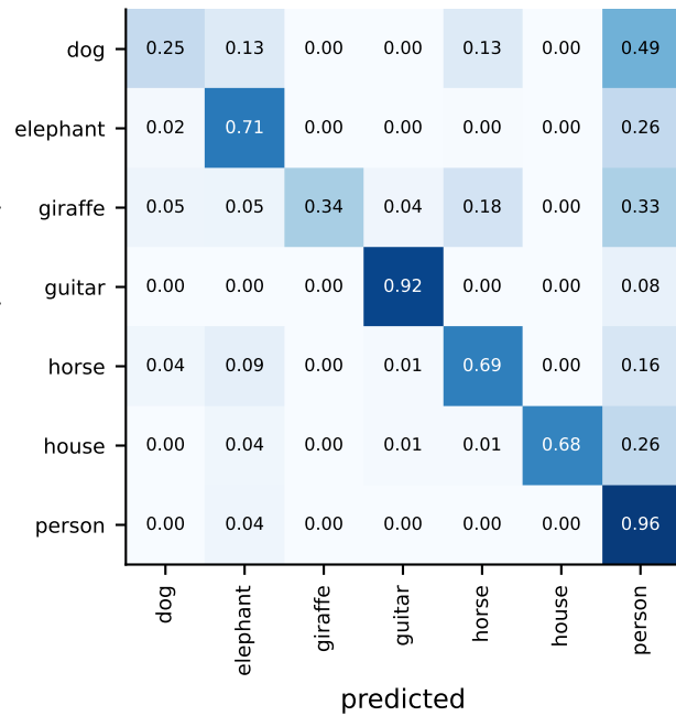
ERM (acc 0.589)
