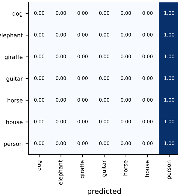
DAN-DG ( \lambda=1 ) (acc 0.041)
