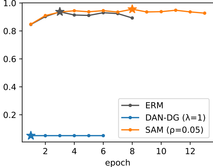
(d) mean source-val macro-F1 ( \star = selected)
