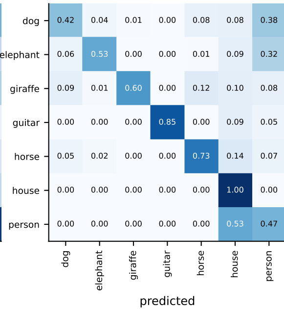
DAN (acc 0.618)
