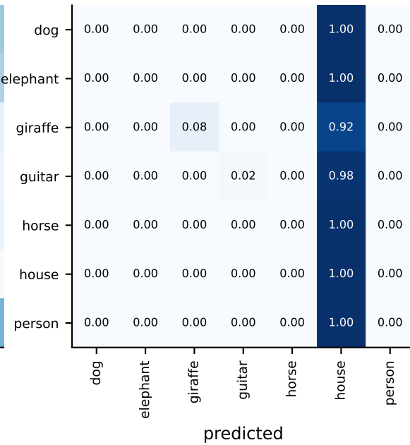
DANN (acc 0.039)
