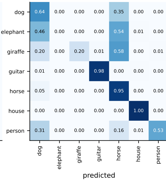
CDAN (acc 0.555)
