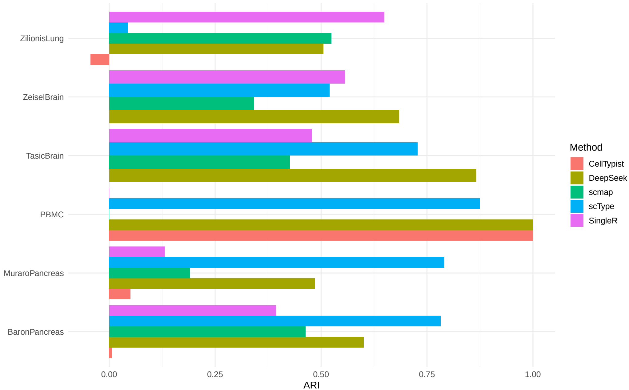
DeepSeekCell benchmark: ARI
