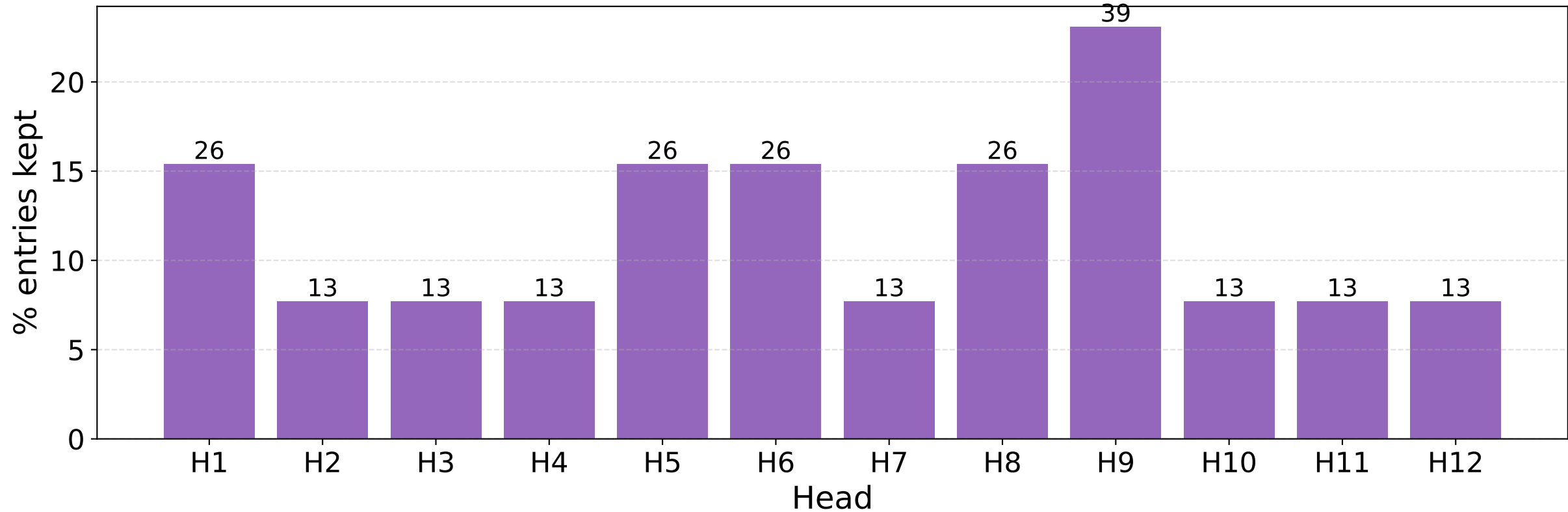
S4 Step 2 — Mask sparsity per head (K=1.0)
