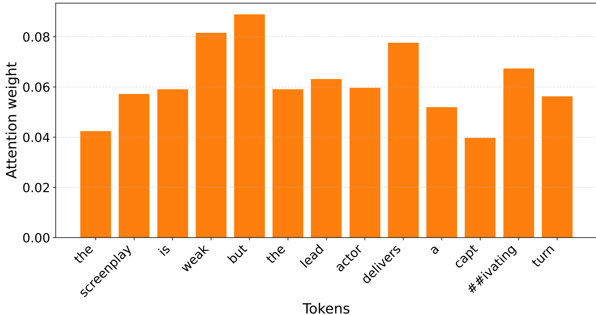
S8 [POS] — Raw attention CLS row (filtered tokens)
