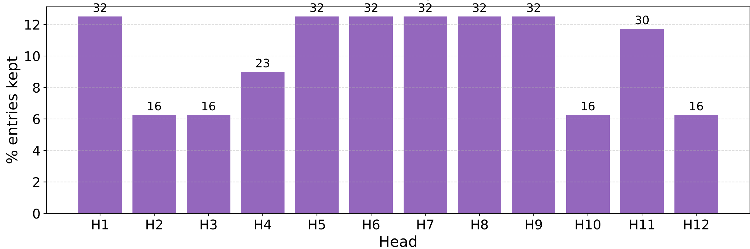
S9 Step 2 — Mask sparsity per head (K=1.0)
