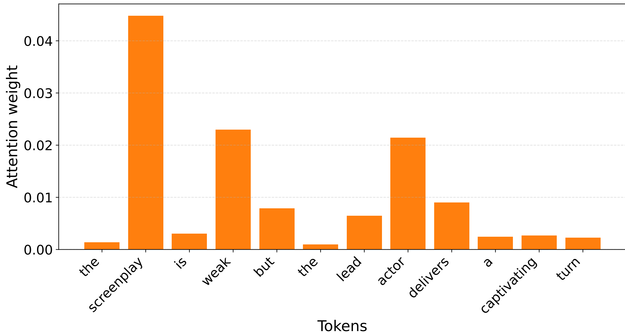
S8 [POS] — Raw attention EOS row (filtered tokens)
