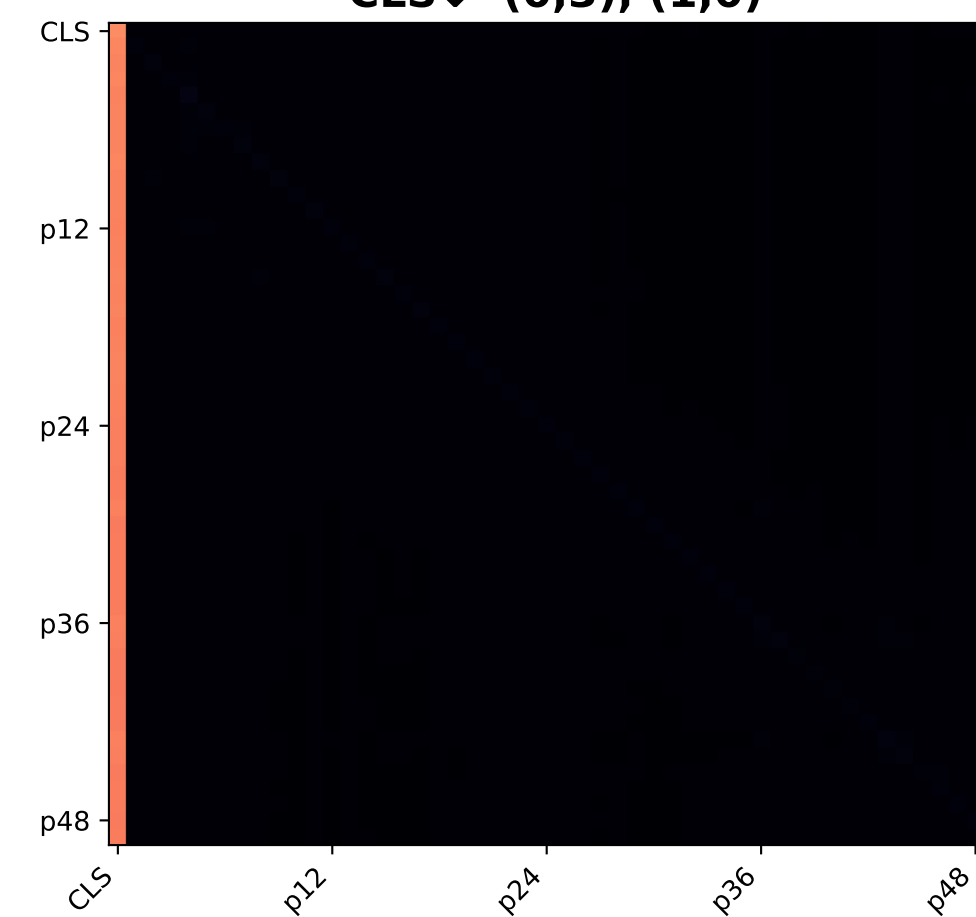
Layer 8 CLS↓ (0,3), (1,0)
