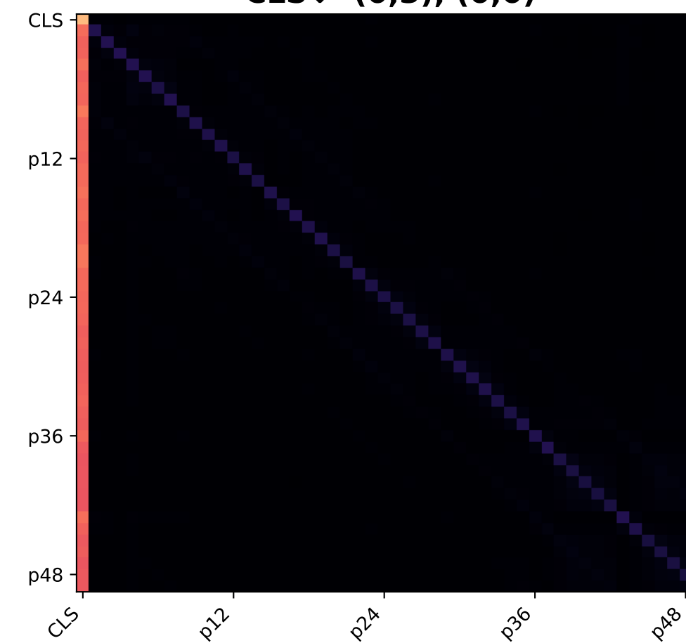
Layer 4 CLS↓ (0,3), (0,0)
