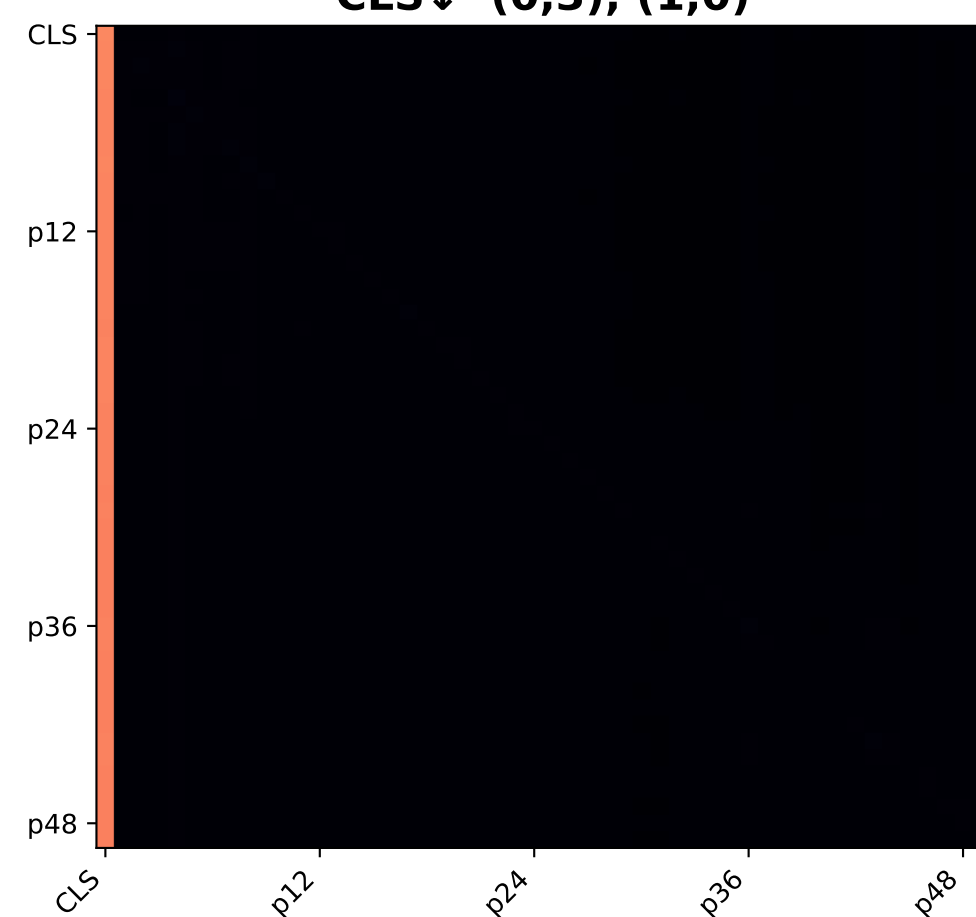
Layer 10 CLS ↓ (0,3), (1,0)
