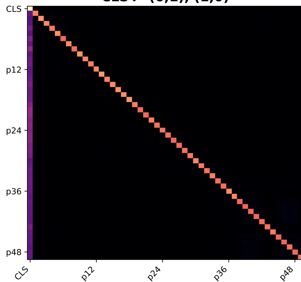
Layer 1 CLS↓ (6,1), (1,0)
