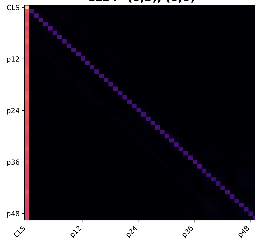
Layer 3 CLS↓ (0,3), (0,0)
