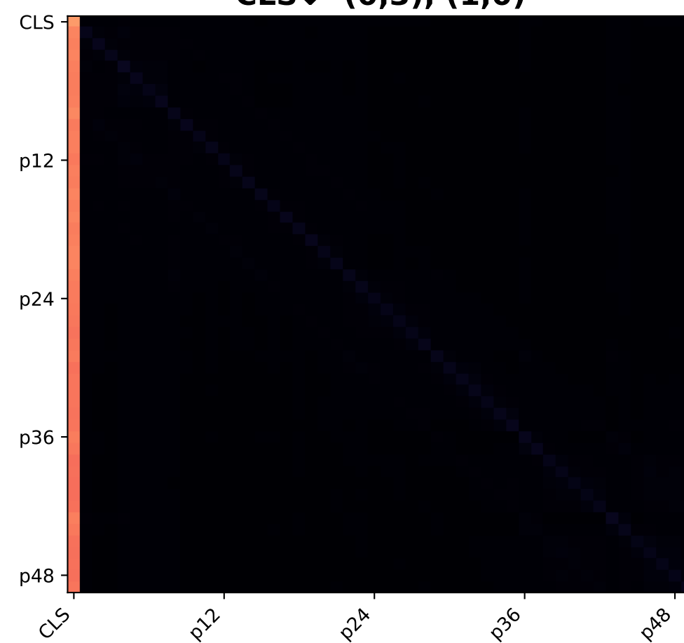
Layer 6 CLS↓ (0,3), (1,0)
