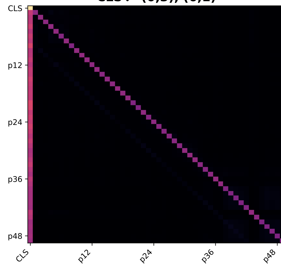
Layer 2 CLS↓ (0,3), (6,1)
