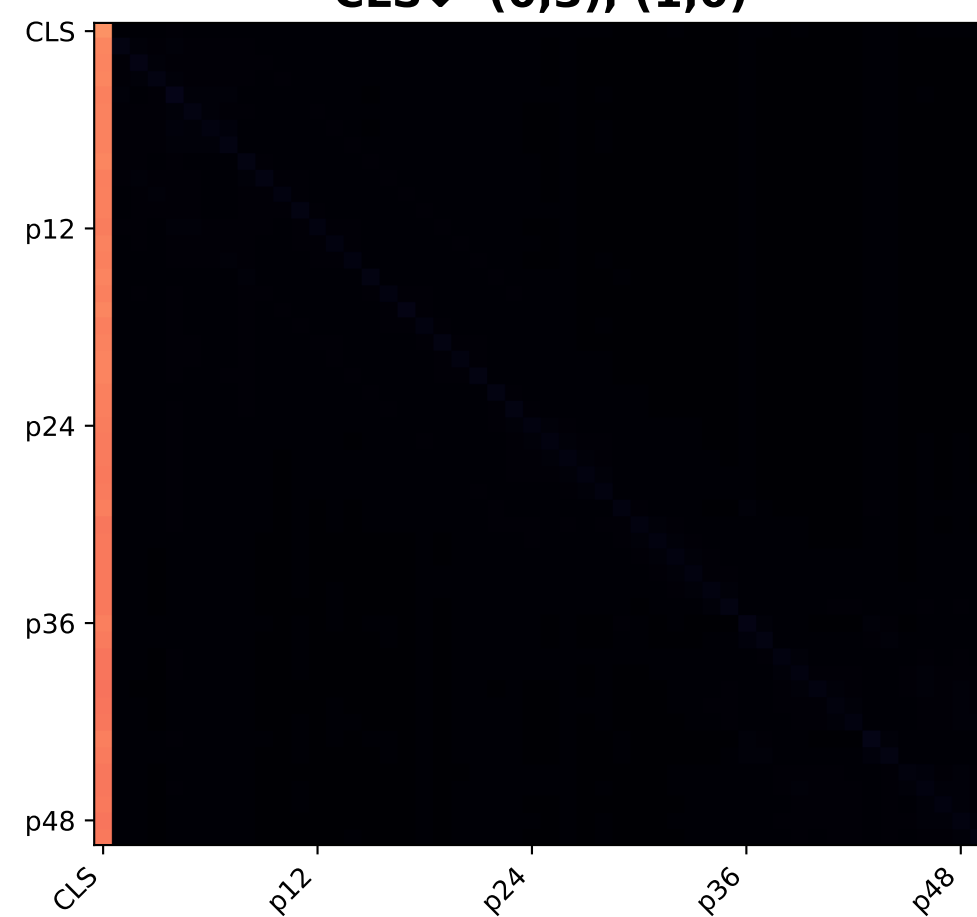
Layer 7 CLS↓ (0,3), (1,0)
