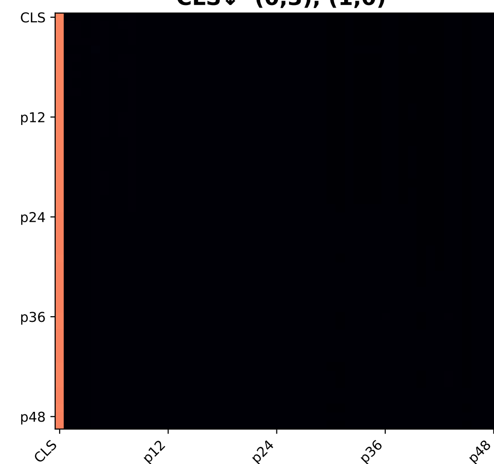
Layer 12 CLS↓ (0,3), (1,0)
