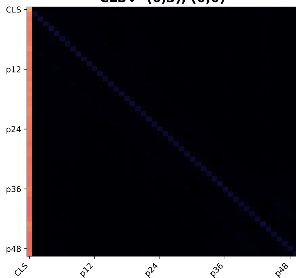
Layer 5 CLS ↓ (0,3), (0,0)
