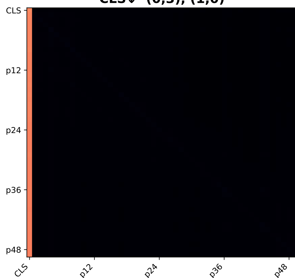
Layer 9 CLS↓ (0,3), (1,0)
