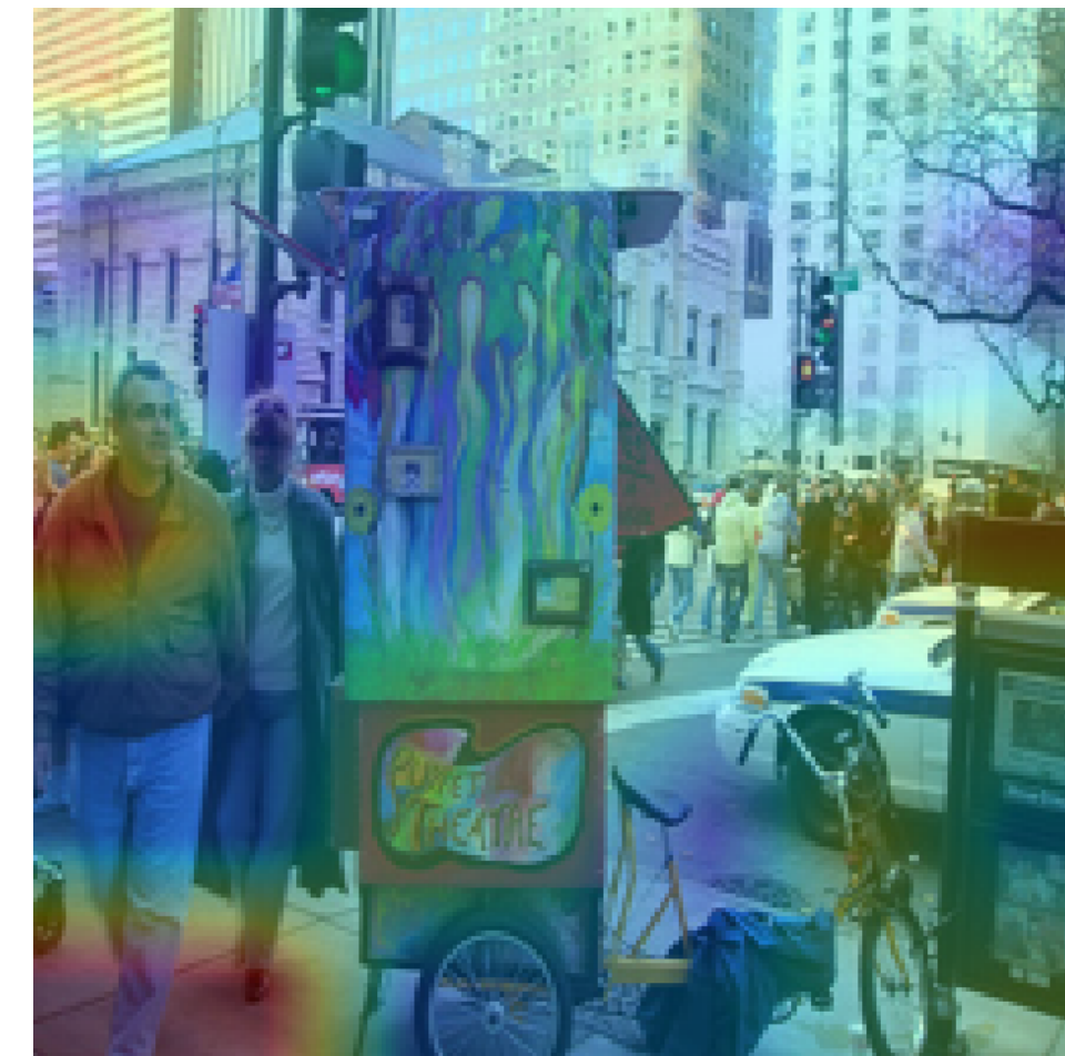
Layer 12
