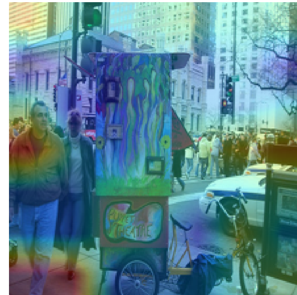
Layer 11
