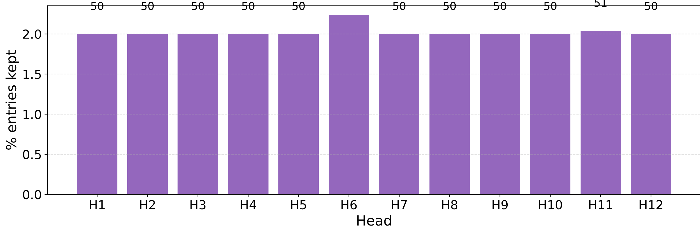
27782020_4dab210360 Step 2 56 — Mask sparsity per head (K=0.0)
