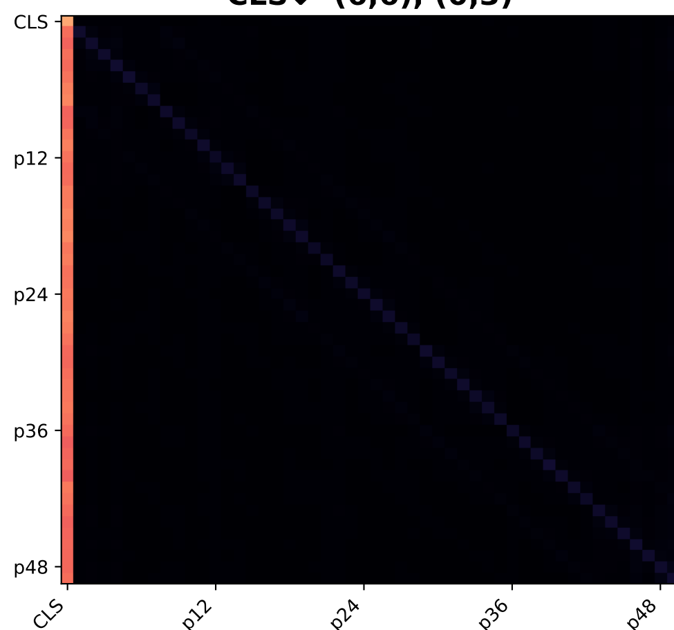
Layer 5 CLS↓ (6,6), (0,3)
