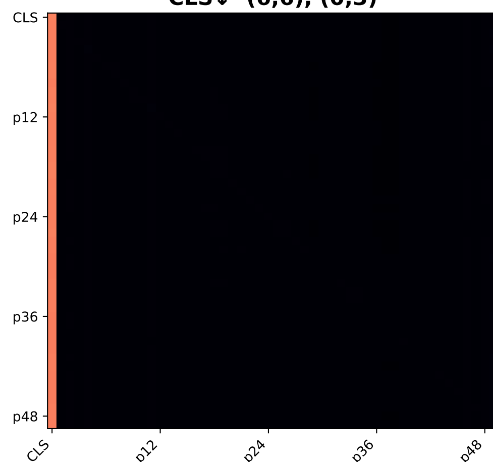
Layer 11 CLS↓ (6,6), (0,3)
