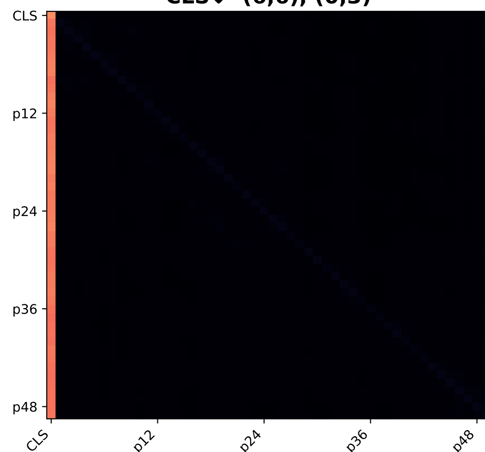
Layer 7 CLS↓ (6,6), (0,3)
