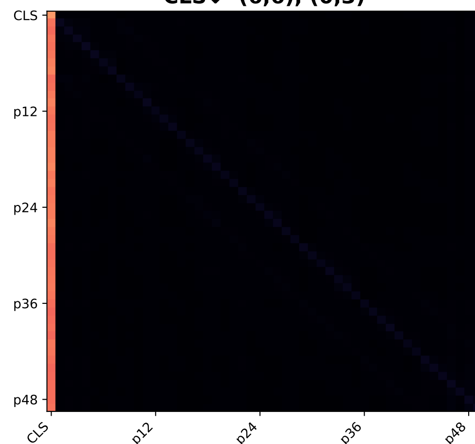
Layer 6 CLS↓ (6,6), (0,3)
