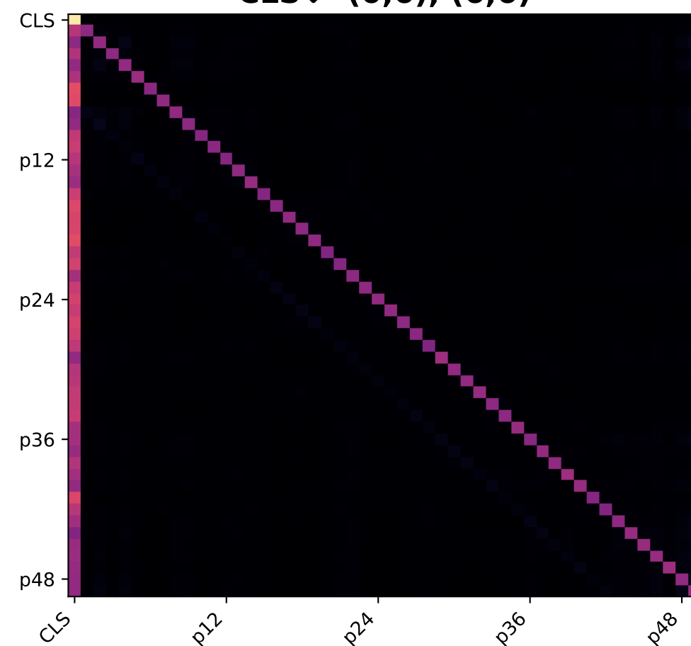
Layer 2 CLS↓ (0,6), (6,6)
