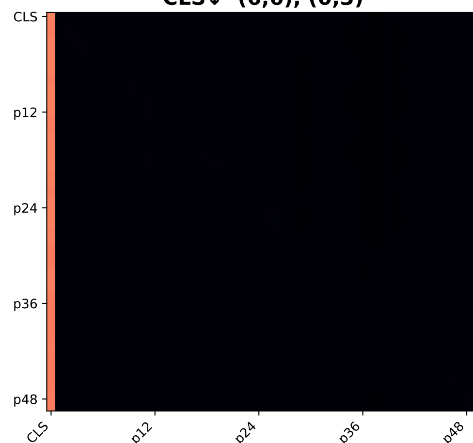
Layer 10 CLS ↓ (6,6), (0,3)
