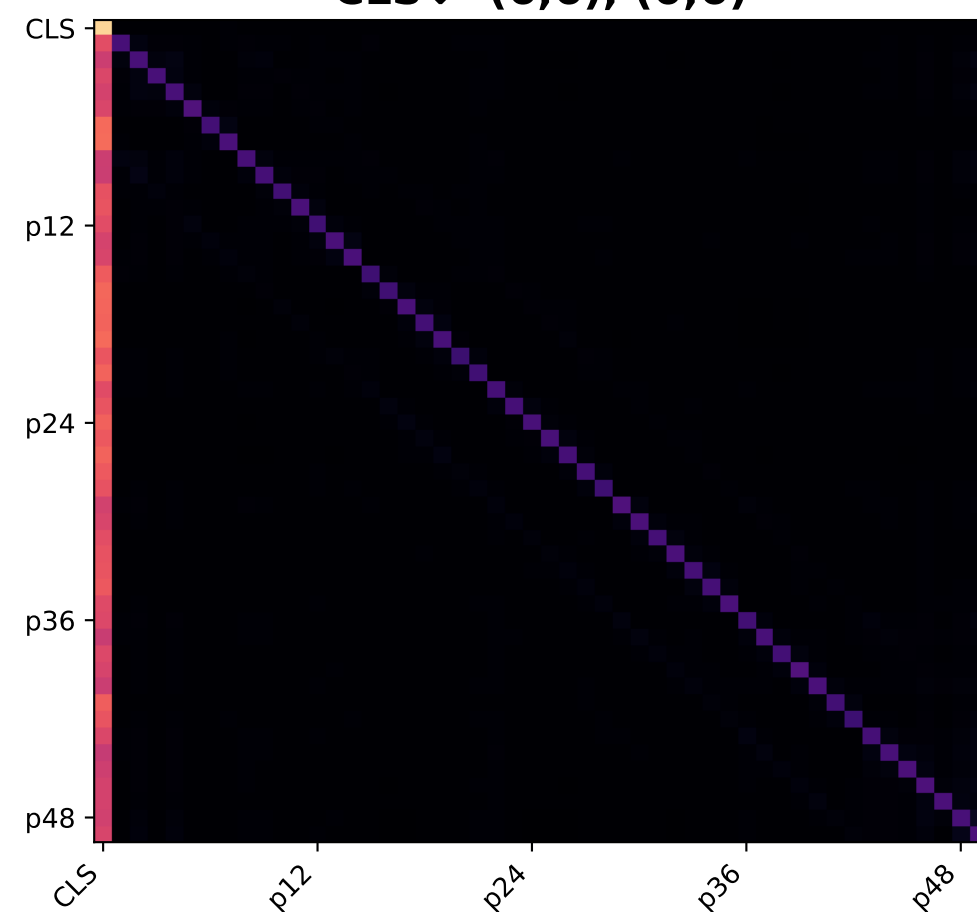
Layer 3 CLS↓ (6,6), (0,6)
