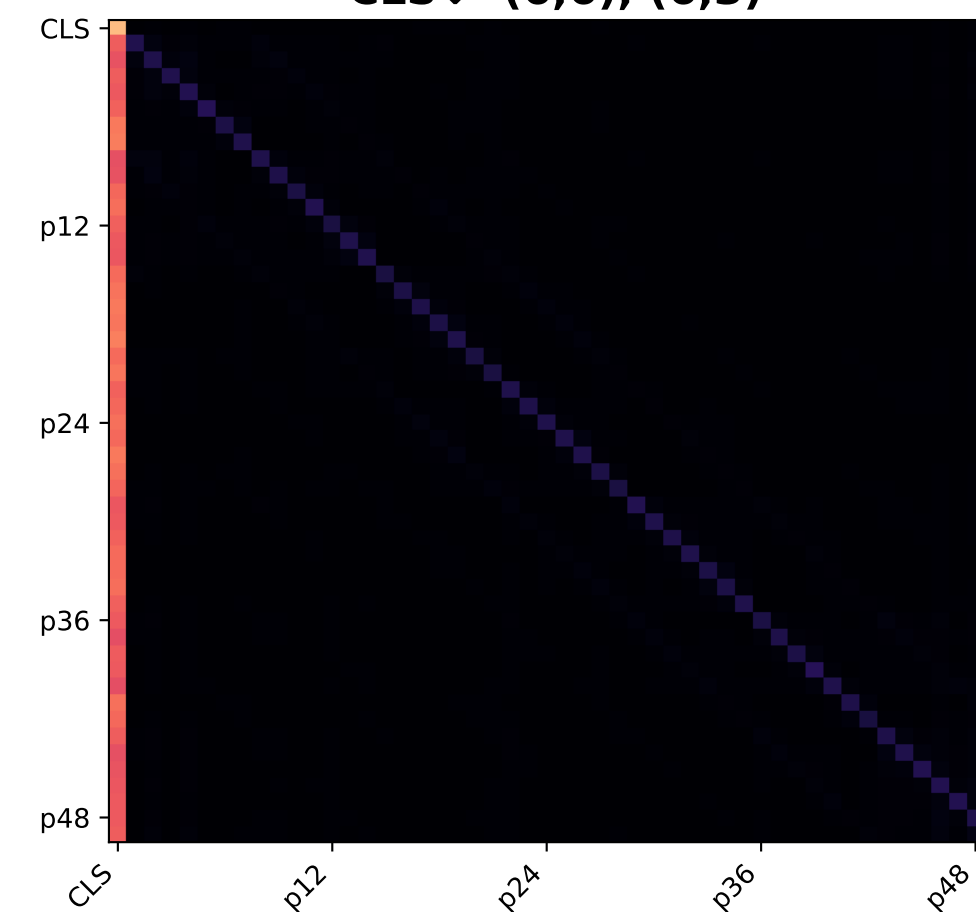
Layer 4 CLS↓ (6,6), (6,3)
