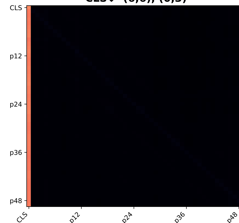
Layer 8 CLS↓ (6,6), (0,3)
