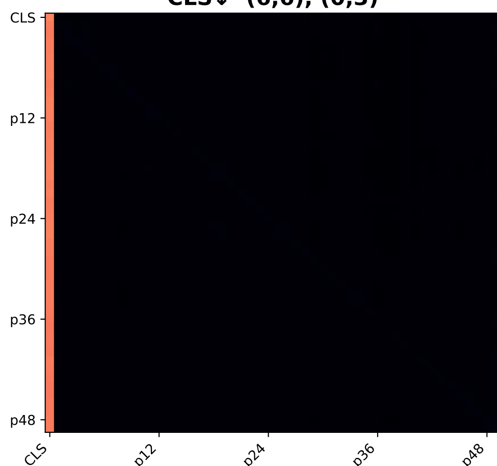
Layer 9 CLS↓ (6,6), (0,3)
