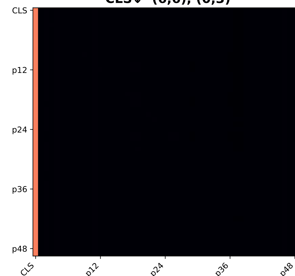
Layer 12 CLS↓ (6,6), (0,3)
