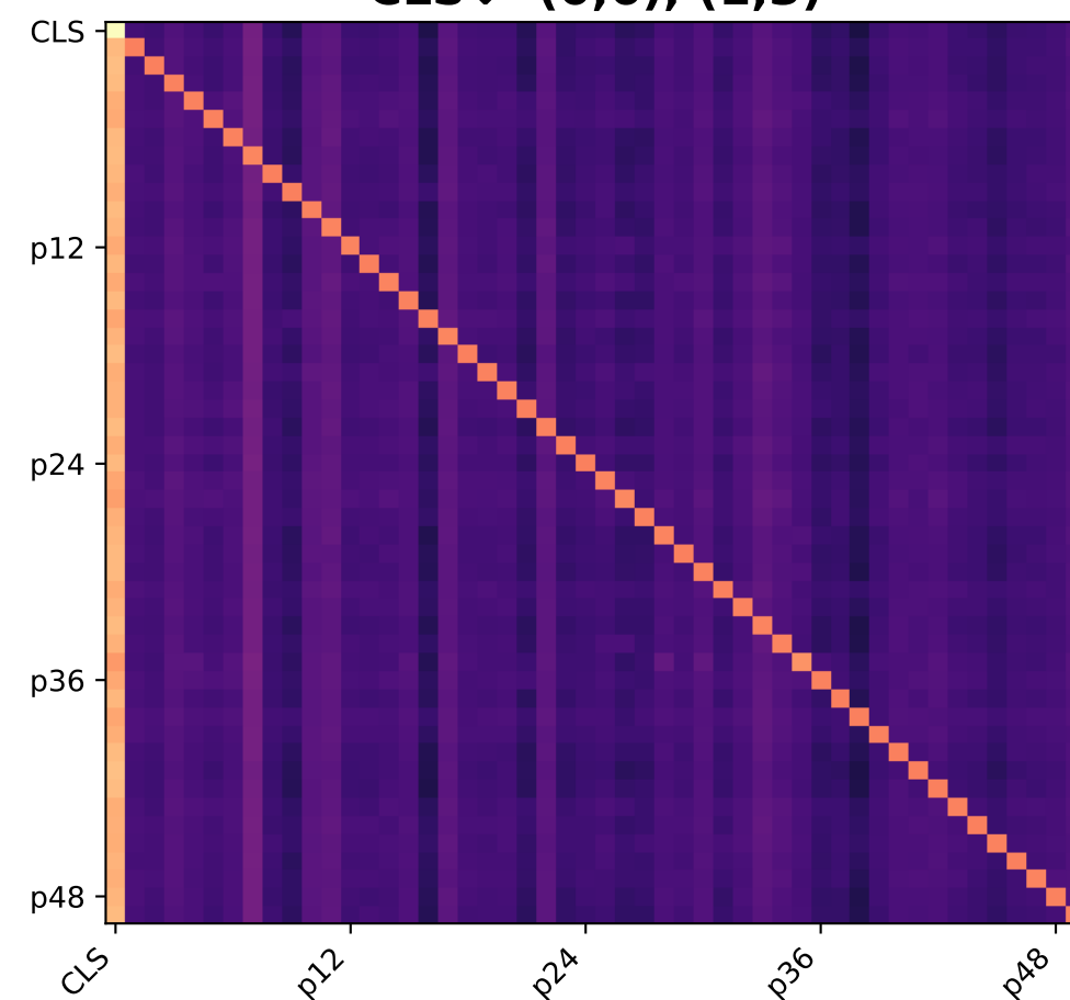
Layer 2 CLS↓ (0.6). (1.3)
