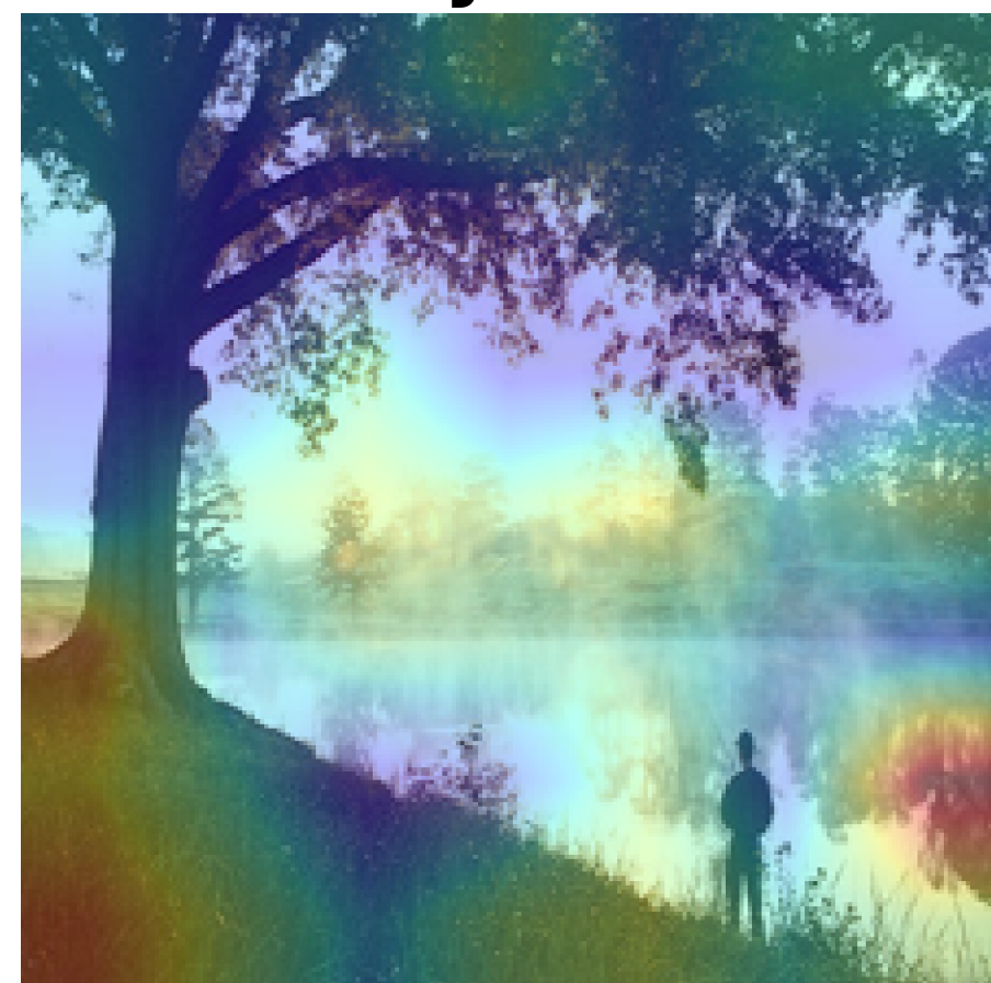
Layer 9
