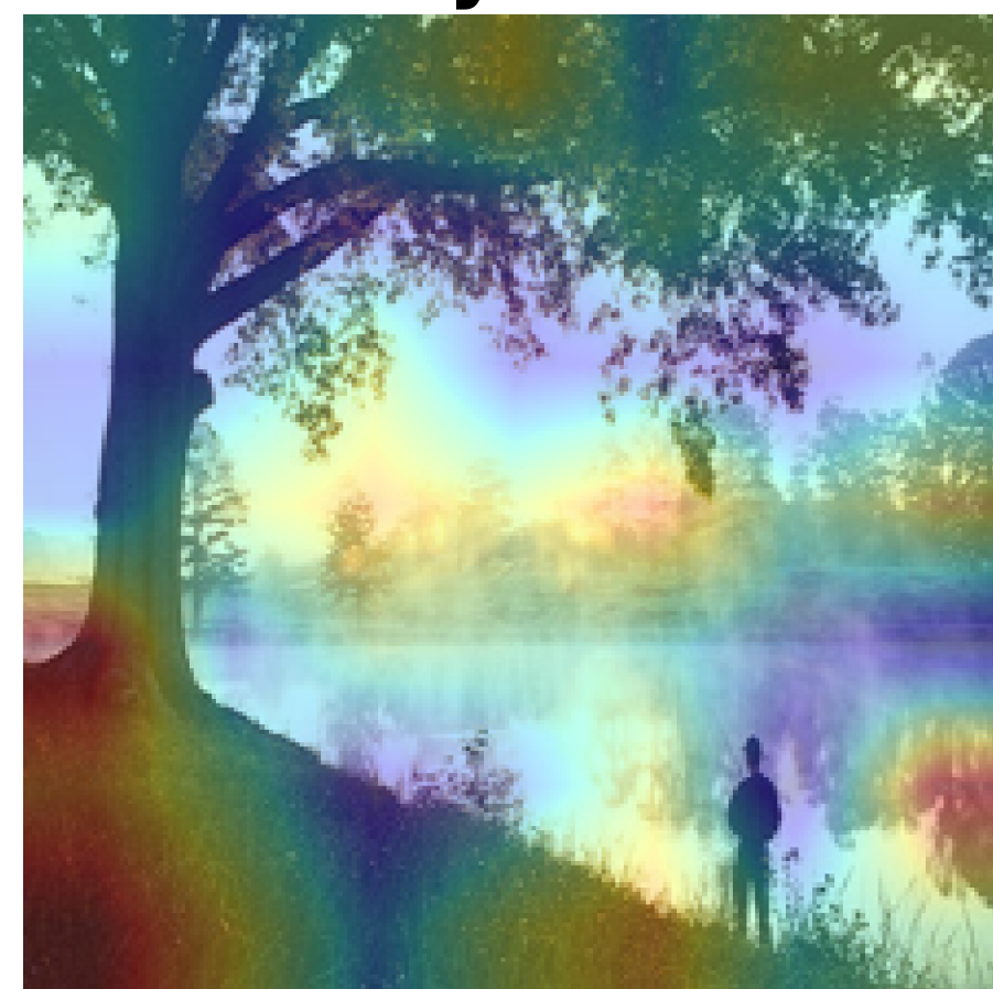
Layer 6
