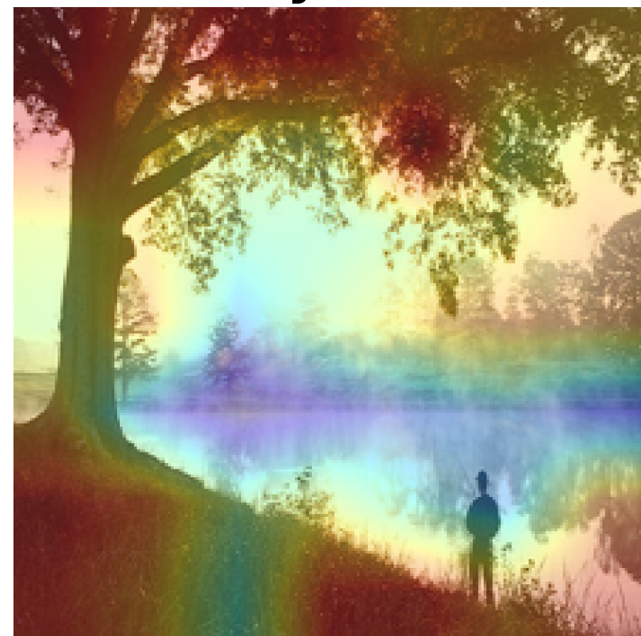
Layer 1
