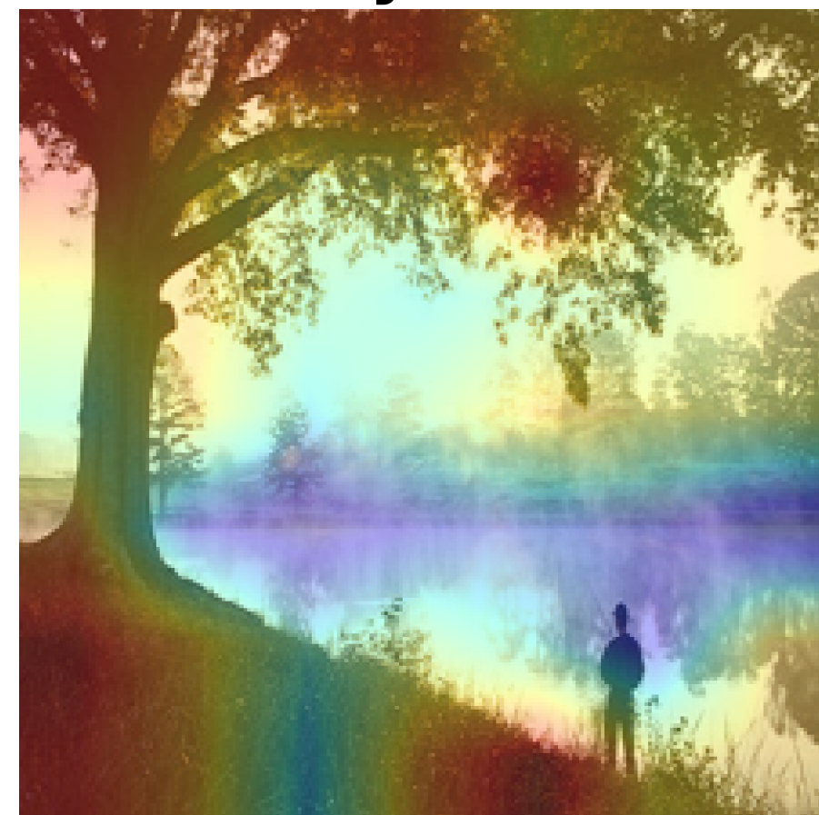
Layer 2
