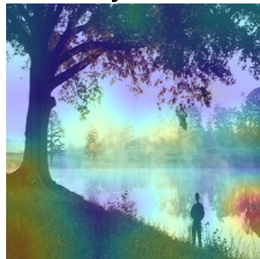
Layer 10
