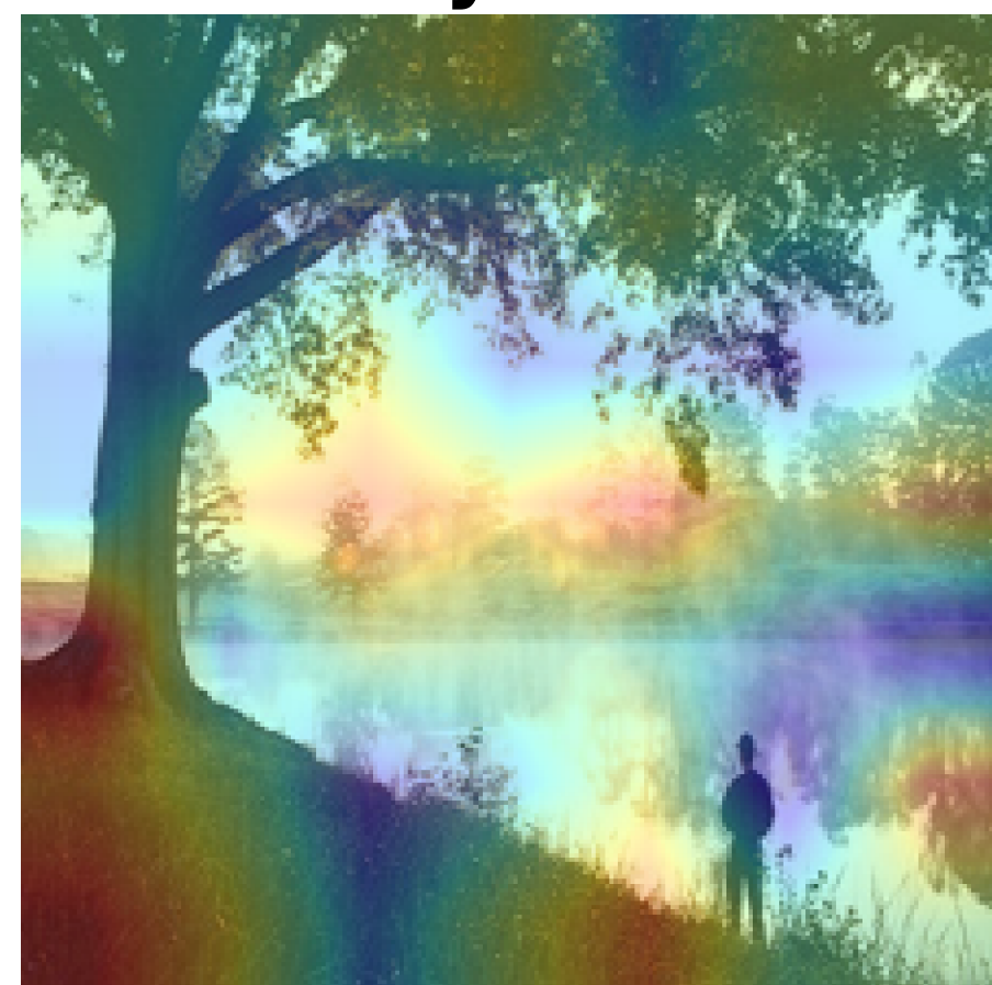
Layer 5
