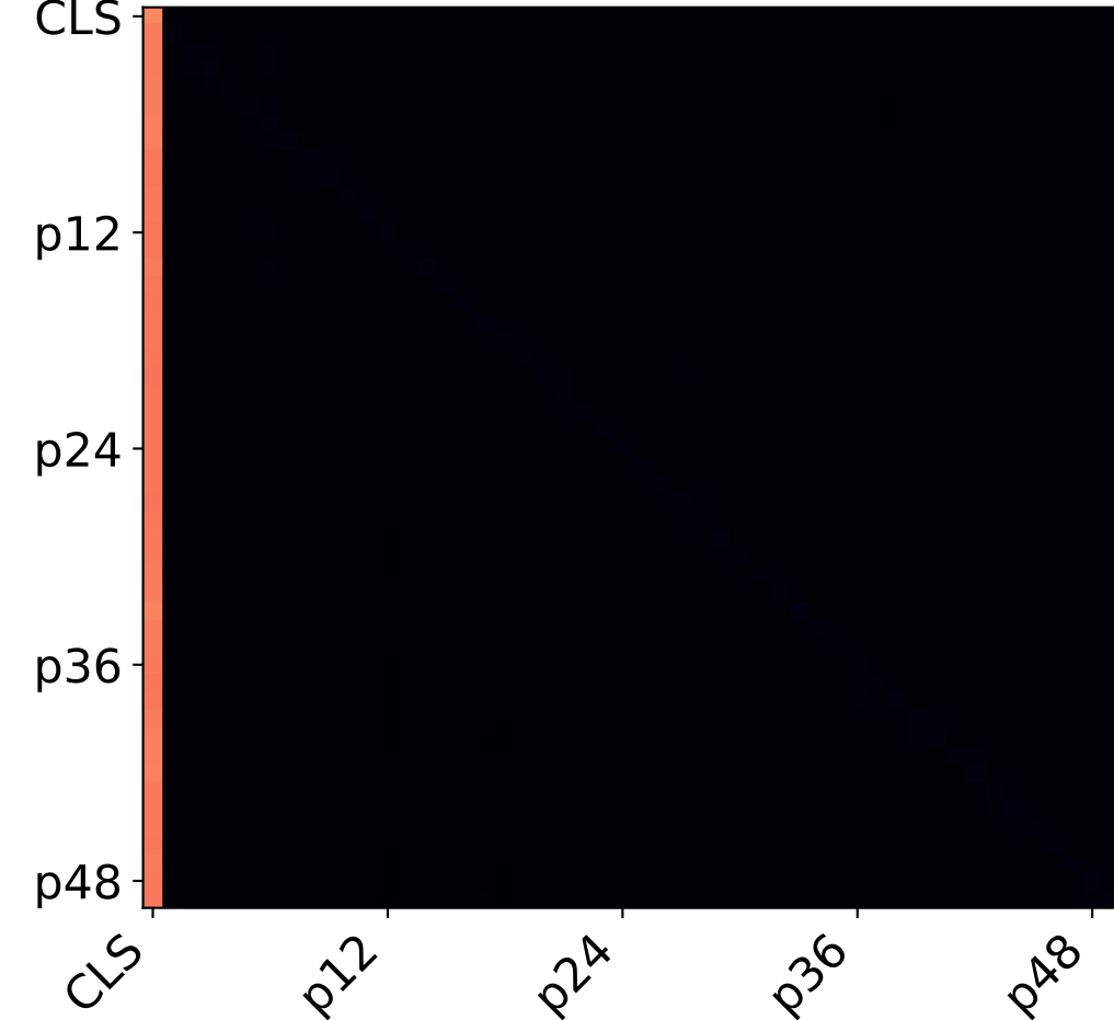
Layer 12 CLS↓ (4,4), (0,5)
