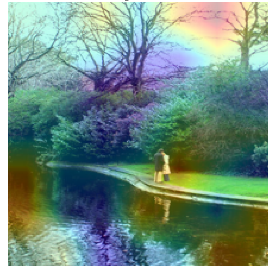
Layer 8
