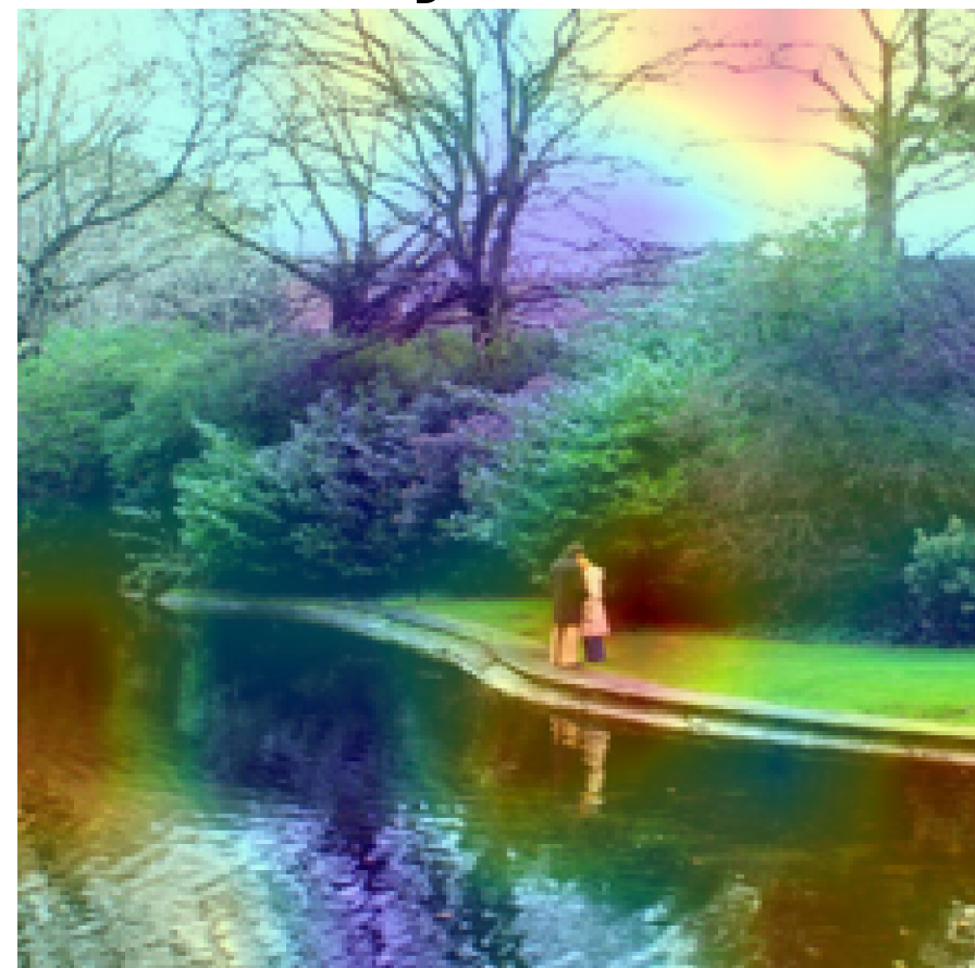
Layer 10
