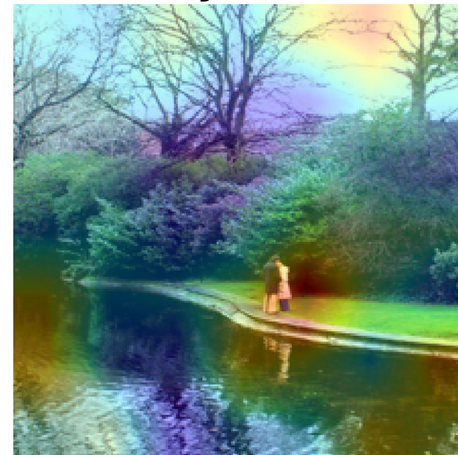
Layer 12
