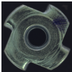
Anomalous input
