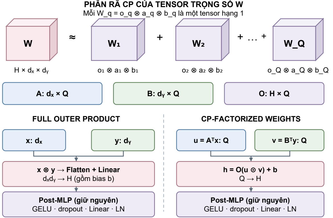
Hình 3.5: Khối 3D biểu diễn tensor trọng số \mathcal{W} \in \mathbb{R}^{d_h \times d_x \times d_y} và tổng các tensor rank-one trong CP; đây là phân rã trọng số, không phải dữ liệu bệnh nhân. Forward dùng hai phép chiếu rank Q , tích Hadamard và phép chiếu output, không dựng \mathcal{W} hay activation outer-product. Phiên bản CP đủ ba pair có low dimensions MR/MC/RC là 32 \times 32 , 32 \times 16 , 32 \times 16 và ranks 8/8/4; post-MLP giữ nguyên.
