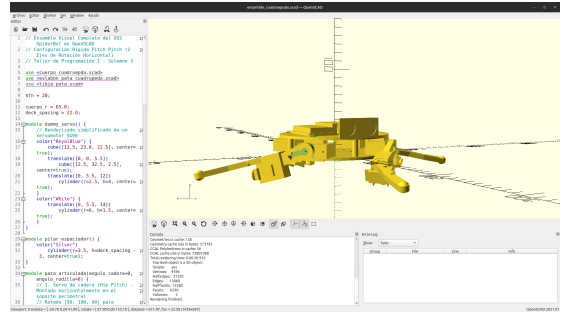
Ensamble definitivo modular en OpenSCAD
