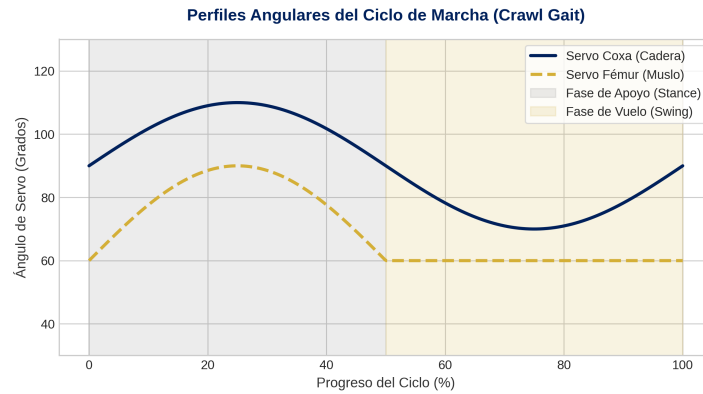
Figura 4: Simulación de la locomoción Crawl Gait con los perfiles angulares asíncronos por articulación.
