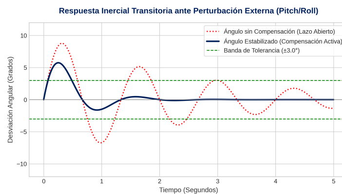
Figura 3: Respuesta transitoria simulada en Python del lazo cerrado de compensación activa de inclinación (Pitch y Roll).
