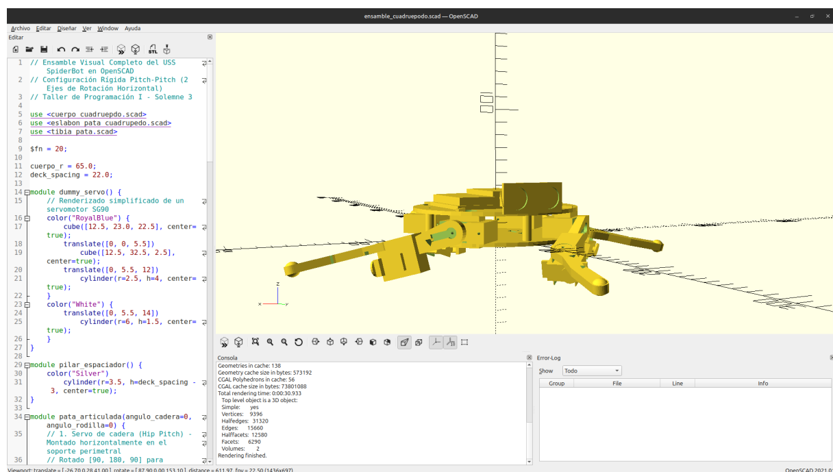
Figura 4: Renderizado y ensamblaje tridimensional completo del USS SpiderBot en el entorno de OpenSCAD.
