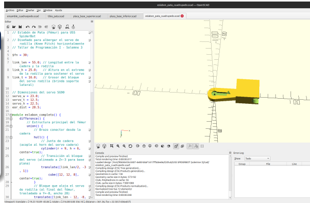
Diseño paramétrico del Eslabón Fémur en OpenSCAD
