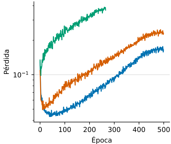
Validación
