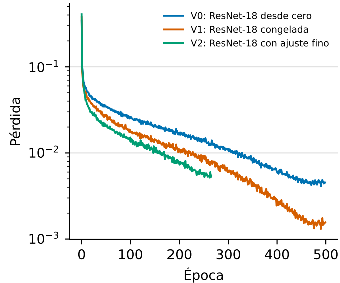
Entrenamiento
