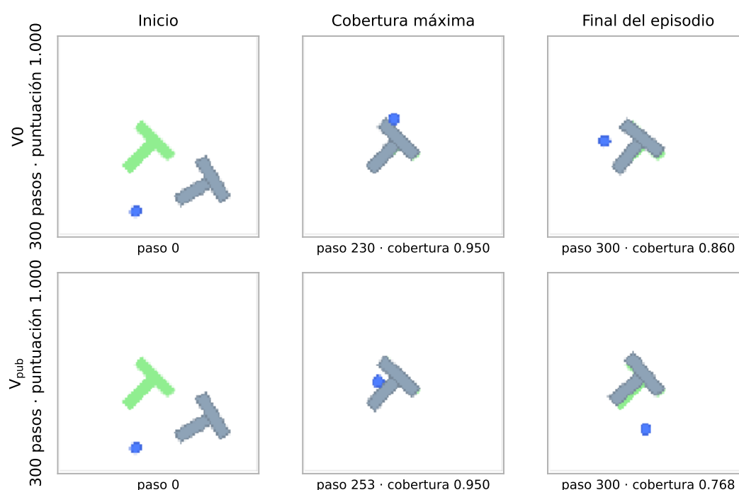
Figura 5. Condición B: la misma condición inicial con la imagen generada por el propio simulador alternativo.
