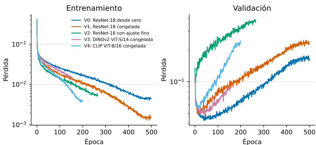
Figura 6. Evolución de las pérdidas de entrenamiento y validación.
