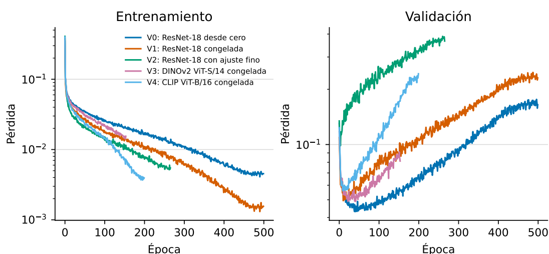
Figura 4. Evolución de las pérdidas de entrenamiento y validación.
