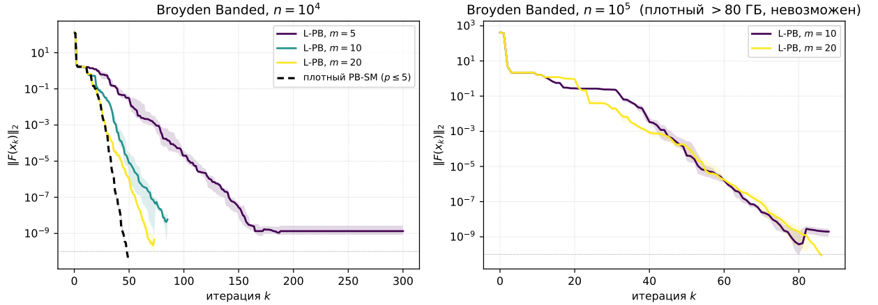
Рисунок 2. Broyden Banded. Медианная траектория \|F(x_k)\|_2 + \text{IQR} по случайным стартам. Слева — n = 10^4 с плотным Projected Broyden-SM ( p \leq 5 , чёрный пунктир) как baseline; справа — n = 10^5 , где плотная форма требует \approx 80 ГБ оперативной памяти и неприменима.
