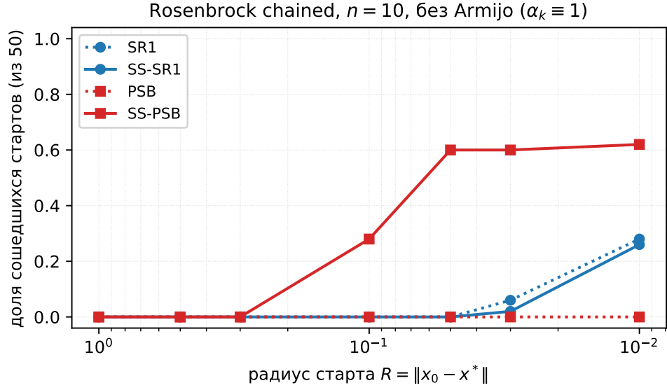
Рисунок 7. Доля сошедшихся стартов (из 50) на Rosenbrock chained, n = 10 , x^* = 1 , против радиуса R = \|x_0 - x^*\| , без backtracking-Армихо. PSB не сходится ни на одном из тестированных радиусов; SS-PSB расширяет область устойчивой сходимости при умеренно малых R . Прямое визуальное подтверждение нетривиальности (Н4) на невыпуклых задачах.
