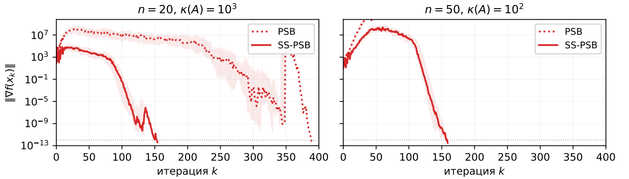
Рисунок 6. Локальная сходимость без Armijo на выпуклой квадратике f(x) = \frac{1}{2} x^\top A x , \|x_0\| = 0.3 , 50 стартов; медиана \|\nabla f(x_k)\| и межквартильный коридор. Слева — режим, где оба обновления сходятся: SS-PSB укорачивает пре-асимптотическую фазу PSB в несколько раз. Справа — режим, где PSB не сходится за бюджет итераций, а SS-PSB сходится: расширение области устойчивого поведения. SR1-семейство опущено: на квадратике SR1 имеет конечную сходимоссть за \leq n + 1 шагов [10], а SS-добавка по rate-invariance (замечание 3.16) её не улучшает.
