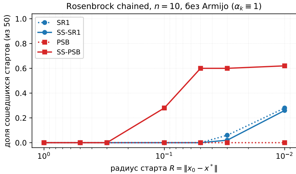
Рисунок 7. Доля сошедшихся стартов (из 50) на Rosenbrock chained, n = 10 , x^* = \mathbf{1} , против радиуса R = \|x_0 - x^*\| , без backtracking-Армихо. PSB не сходится ни на одном из тестируемых радиусов; SS-PSB расширяет область устойчивой сходимости при умеренно малых R . Прямое визуальное подтверждение нетривиальности (H4) на невыпуклых задачах.
