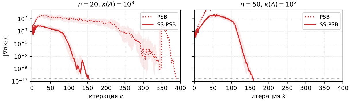
Рисунок 6. Локальная сходимость без Armijo на выпуклой квадратике f(x) = \frac{1}{2}x^\top Ax , \|x_0\| = 0.3 , 50 стартов; медиана \|\nabla f(x_k)\| и межквартильный коридор. Слева — режим, где оба обновления сходятся: SS-PSB укорачивает пре-асимптотическую фазу PSB в несколько раз. Справа — режим, где PSB не сходится за бюджет итераций, а SS-PSB сходится: расширение области устойчивого поведения. SR1-семейство опущено: на квадратике SR1 имеет конечную сходимость за \leq n + 1 шагов [10], а SS-добавка по rate-invariance (замечание 3.16) её не улучшает.
