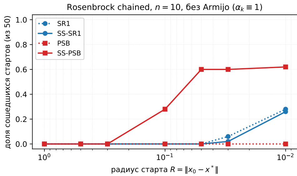
Рисунок 7. Доля сошедшихся стартов (из 50) на Rosenbrock chained, n = 10 , x^* = \mathbf{1} , против радиуса R = \|x_0 - x^*\| , без backtracking-Армихо. PSB не сходится ни на одном из тестируемых радиусов; SS-PSB расширяет область устойчивой сходимости при умеренно малых R . Прямое визуальное подтверждение нетривиальности (Н4) на невыпуклых задачах.
