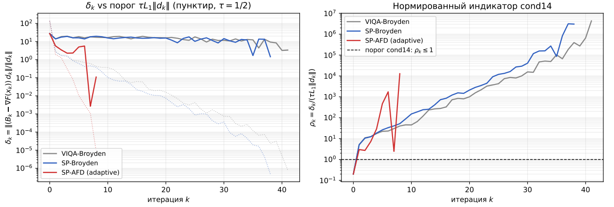
Рисунок 10. Эмпирическая проверка (56) на cubic-monotone, (n, \kappa, \varepsilon) = (30, 20, 1, 5) , seed = 0. Слева: \delta_k = \|(B_k - \nabla F(x_k))d_k\| / \|d_k\| (сплошные) и порог \tau L_1 \|d_k\| (пунктиры того же цвета). Справа: нормированный индикатор \rho_k = \delta_k / (\tau L_1 \|d_k\|) ; условие (56) выполнено iff \rho_k \leq 1 (горизонтальная чёрная пунктирная линия). VIQA-Broyden и SP-Broyden нарушают условие систематически ( \rho_k \rightarrow 10^6 ); SP-AFD-adaptive в активной фазе подавляет \rho_k ниже за счёт refinement-loop.
