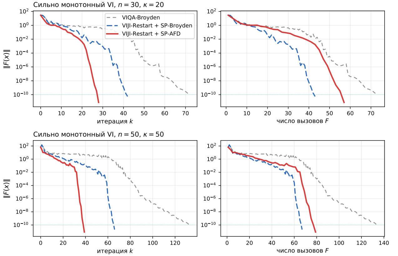
Рисунок 6. Сходимость трёх квазиньютоновских методов на сильно монотонной VI с кубической нелинейностью. Слева — по итерациям, справа — по числу вызовов F . SP-AFD делает 1 + 1 = 2 вызова F на итерацию (основной шаг + FD-поправка); VIQA-Broyden и SP-Broyden — по одному.
