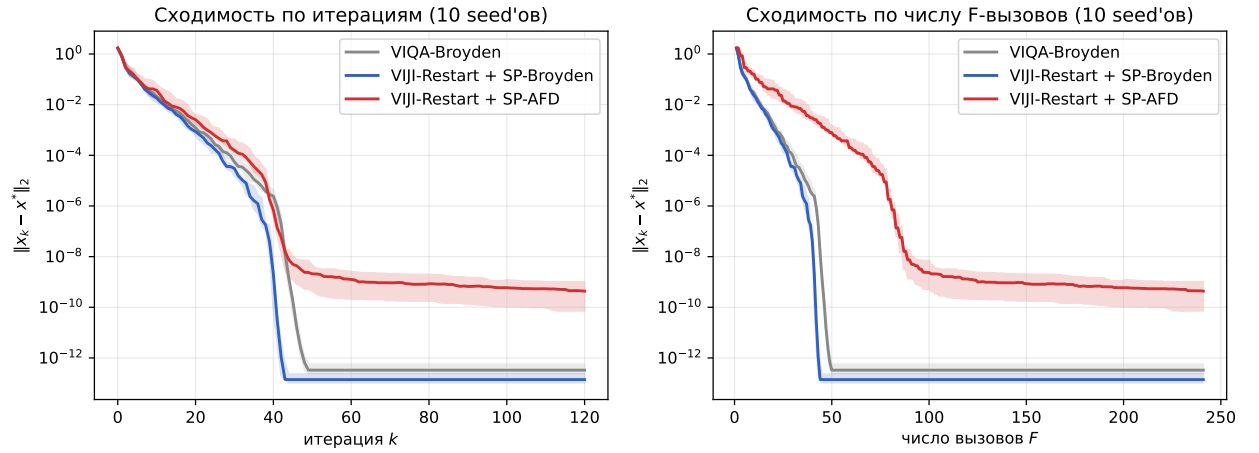
Рисунок 7. Сходимость трёх методов на сильно монотонной VI с кубической нелинейностью, 10 независимых seed'ов. Слева — по итерациям, справа — по числу F -вызовов. Сплошная линия — медиана, заливка — межквартильный размах (25/75%). Конфигурация (n, \kappa, \varepsilon) = (30, 20, 1, 5) , \mu = 1 , L_1 \sim 6\varepsilon ; стартовая точка x_0 = x^* + \mathcal{N}(0, 0,09) \cdot \mathbf{1} . Детали воспроизведения — скрипт run_seeds.py в репозитории SP-Broyden.
