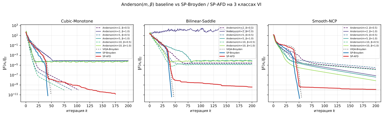
Рисунок 12. Anderson( m, \beta )-baseline (Walker–Ni 2011 со residual-safeguard) vs VIQA-Broyden / SP-Broyden / SP-AFD на трёх классах VI. Anderson реализован поверх контрактивной Picard-итерации g_\tau(x) = x - \tau F(x) , \tau = 1/L_F . Тестируются все комбинации m \in \{2, 5, 10\} , \beta \in \{1/2, 1\} . На всех трёх задачах SP-Broyden / VIQA-Broyden достигают машинной точности ( \leq 10^{-11} ) за 43–55 итераций, тогда как лучшие конфигурации Anderson останавливаются на плато 10^{-5} – 10^{-9} к 200 итерациям.
