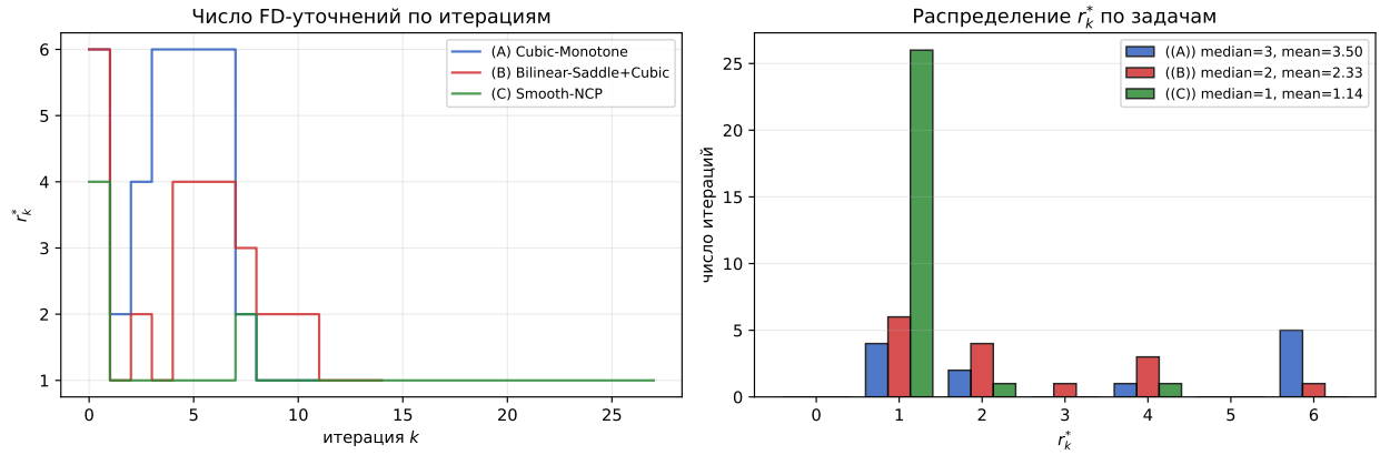
Рисунок 11. Число FD-уточнений r_k^* для SP-AFD-adaptive (триггер cond14 с \tau = 1/2 , r_{\max} = 6 ). Слева — траектория r_k^* vs k для трёх задач; справа — гистограмма r_k^* . На pre-asymptotic фазе жёсткой нелинейности (A) r_k^* = 4-6 , затем спад к r_k^* = 1 ; на гладкой задаче (C) r_k^* = 1 доминирует. Прямое эмпирическое подтверждение proposition 4.3.
