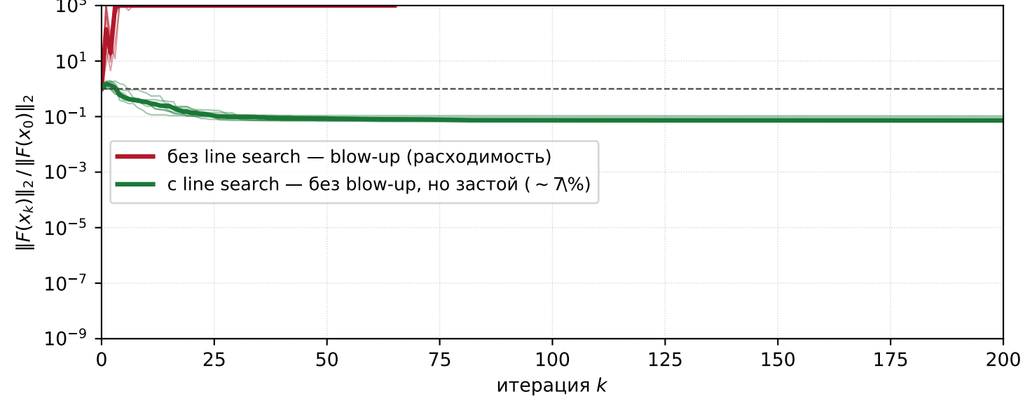
Глобализация убирает blow-up, но не доводит до корня (merit-минимум): Broyden Tridiagonal, d \approx 1.5
