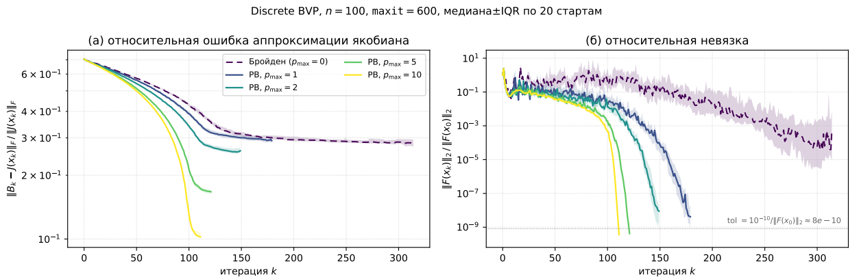
Рисунок 1. Discrete BVP, n = 100 , \|F\|_2 \leq 10^{-10} , \text{maxit} = 600 , 20 случайных стартов; медиана \pm IQR. (а) относительная ошибка якобиана \|B_k - J(x_k)\|_F / \|J(x_k)\|_F для всех p_{\max} остаётся ограниченной — эмпирическая верификация bounded deterioration (17). (б) относительная невязка \|F(x_k)\|_2 / \|F(x_0)\|_2 : классический Бroyден ( p_{\max} = 0 ) за отведённый бюджет не достигает \text{tol} ни на одном из 20 стартов, тогда как РВ при p_{\max} \geq 5 устойчиво сходится. Расширение окна не только усиливает проектор \Pi_k в разложении теоремы 2.10, но и переводит метод из режима «ошибка ограничена, сходимости нет» в режим сверхлинейной сходимости.
