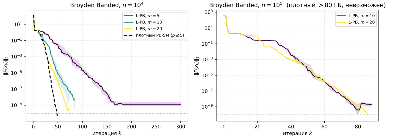
Рисунок 2. Broyden Banded, \|F\|_2 \leq 10^{-10} , backtracking-Армихо c_1 = 10^{-4} . Медианная траектория \|F(x_k)\|_2 + \text{IQR} по случайным стартам x_0 = -0,1 \cdot \mathbf{1} + 0,05 u_i . Слева — n = 10^4 , 8 стартов; плотный Projected Broyden-SM ( p \leq 5 , чёрный пунктир, 3 старта) — baseline. Справа — n = 10^5 , 4 старта; плотная форма требует \approx 80 ГБ оперативной памяти и неприменима.
