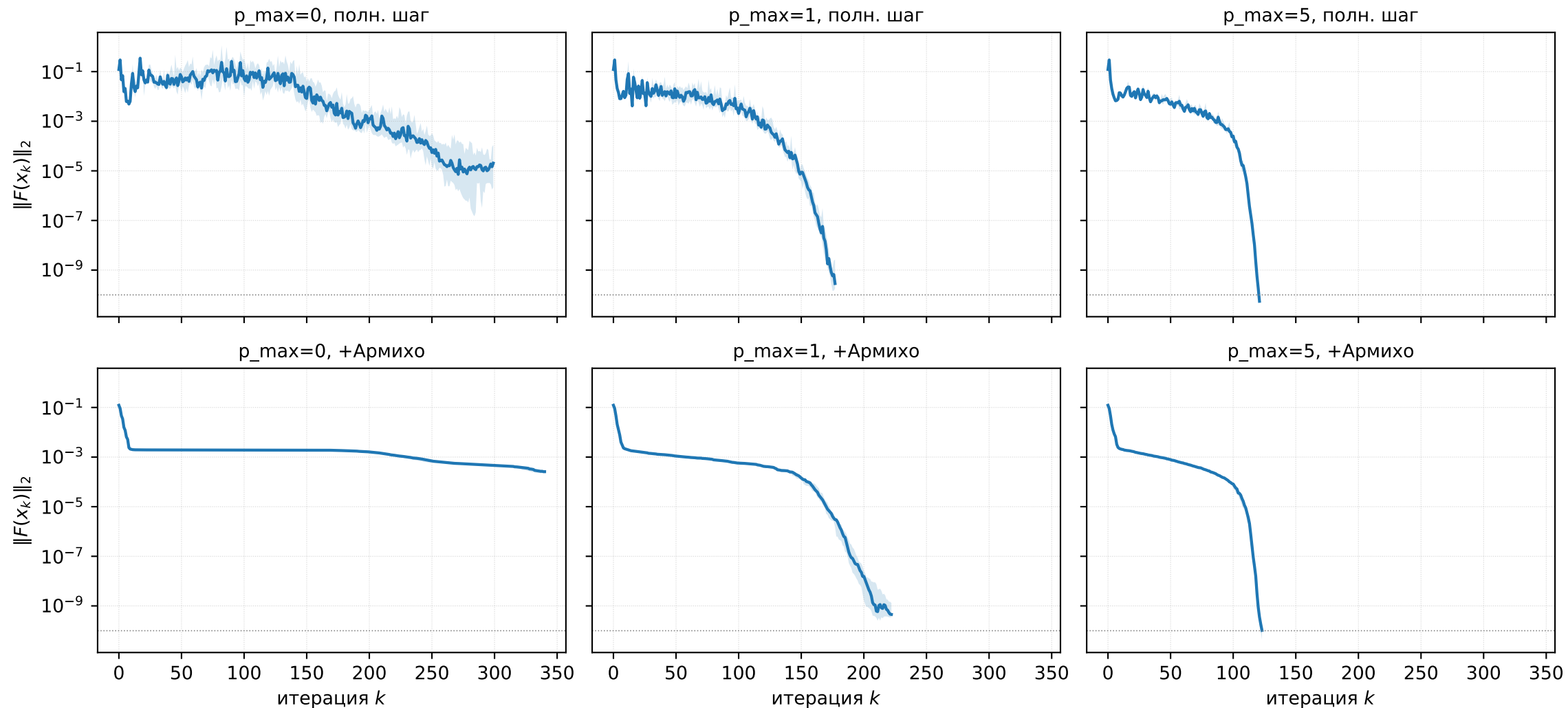
EXP-A: Discrete BVP n = 100 , 20 случайных стартов ( \Delta = 0.05 ); медиана \pm IQR
