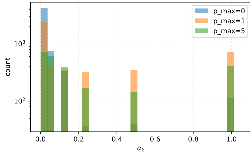
Discrete BVP, n=100, 20 стартов, +Армихо
