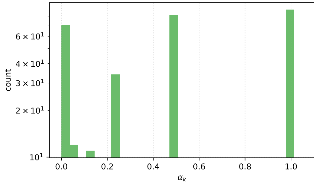
Broyden Banded, n=10^4, L-PB(m=20,p=5), +Армихо
