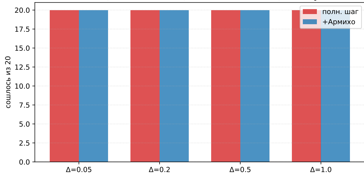
EXP-D: устойчивость РВ( p=5 ) к дальности старта от x_0^{\text{def}}
