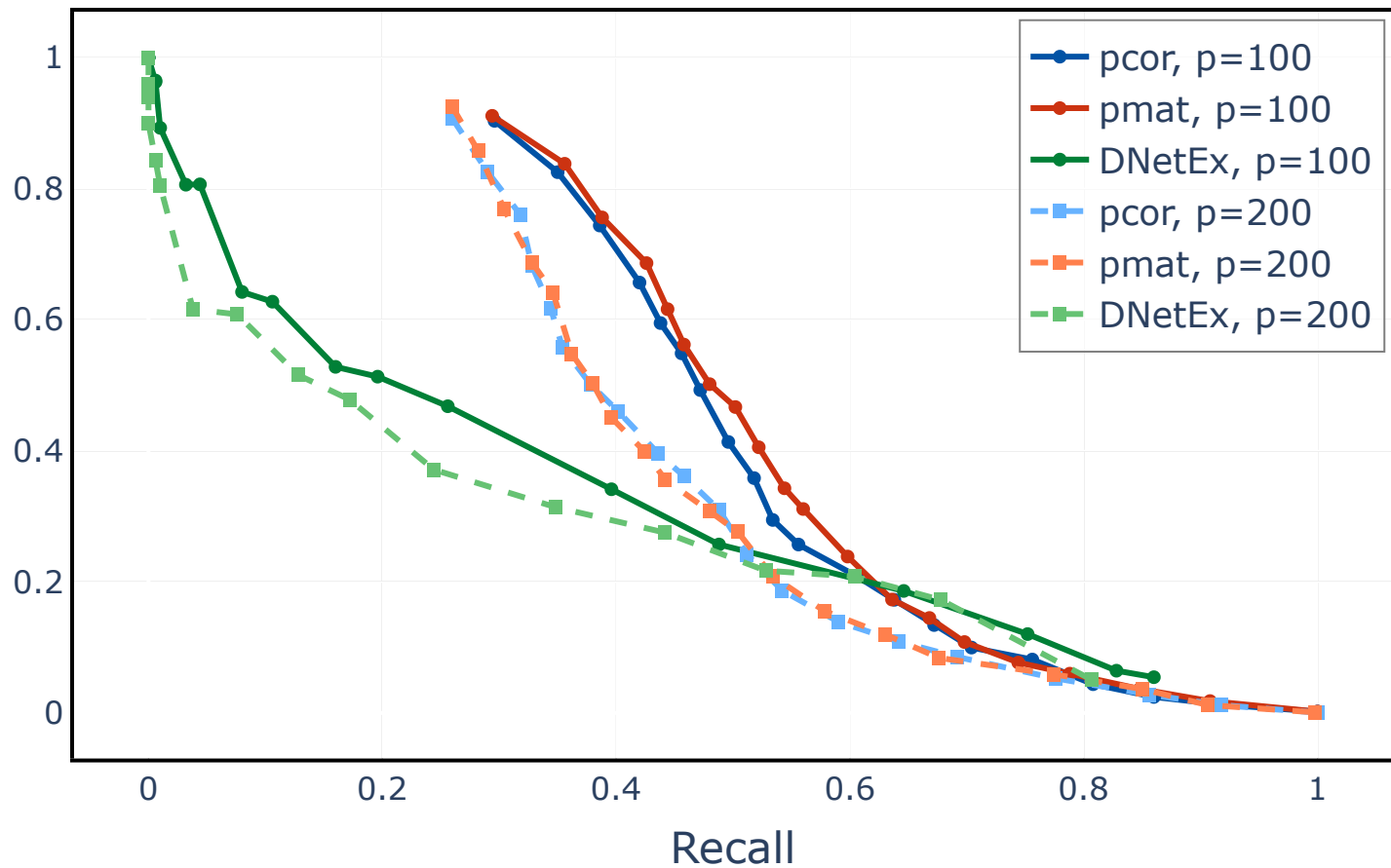
Precision
