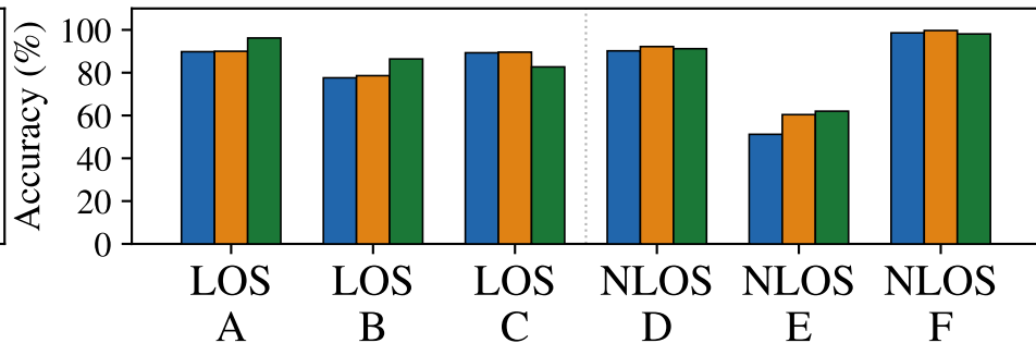
(d) DenseNet
