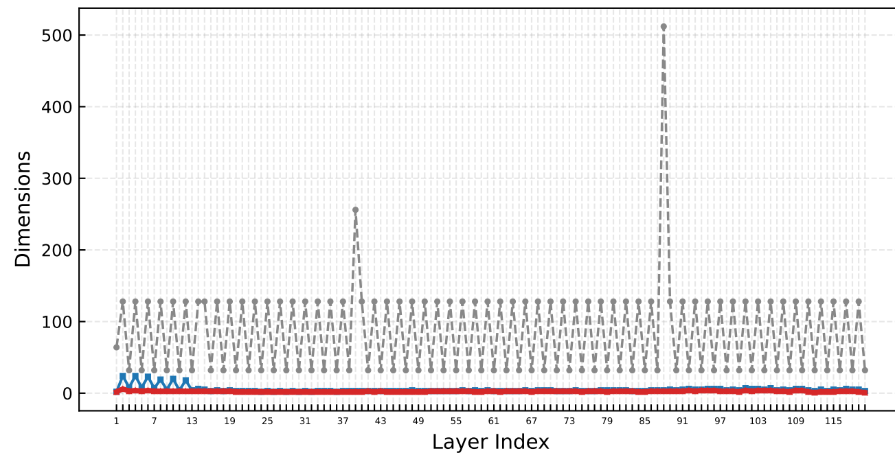
(d) DenseNet
