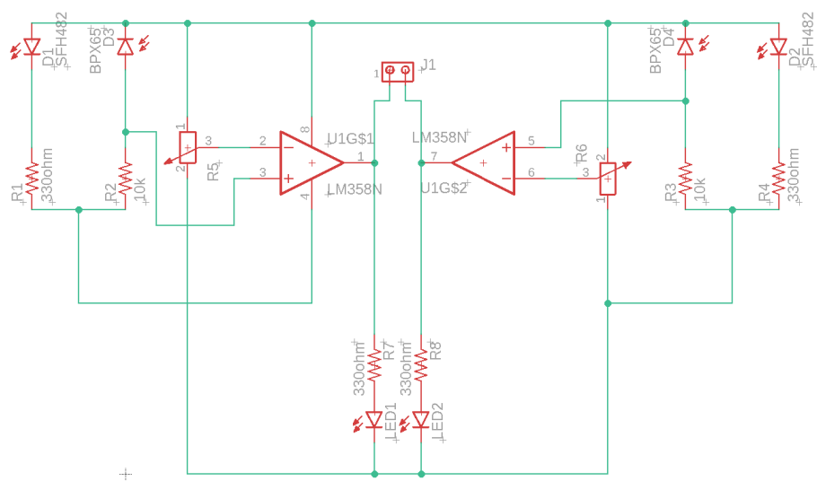
IR Circuit Layout
